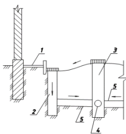
Рис. 8.1. Закрытая ливнесточная система:
