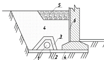
Рис. 8.2. Пристенный дренаж:
