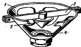
Рис. 11.1. Короткоструйная дождевальная насадка с конусным дефлектором: 1 – конус; 2 – планка; 3 – конусный дефлектор; 4 – выходное отверстие
