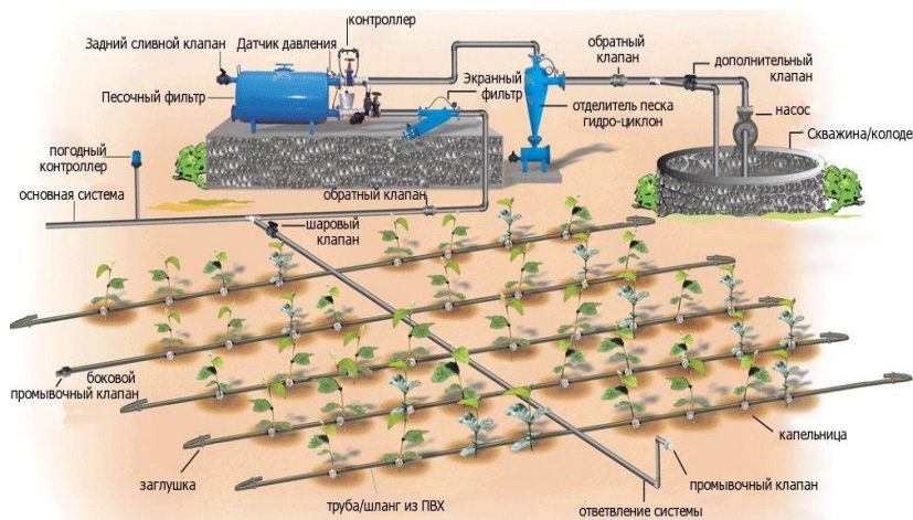
Рис. 11.4. Принципиальная схема системы капельного орошения
