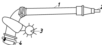
Рис. 11.2. Дальнеструйный дождевальный аппарат: 1 – ствол; 2 – сопло; 3 – механизм привода вращения (гидравлическая турбинка); 4 – присоединительный узел
