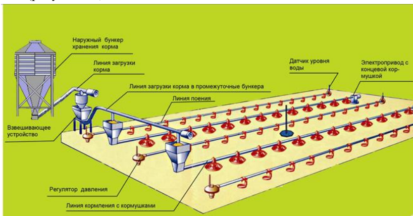
Рисунок .... – Оборудование для напольного содержания бройлеров фирмы Big Dutchman
