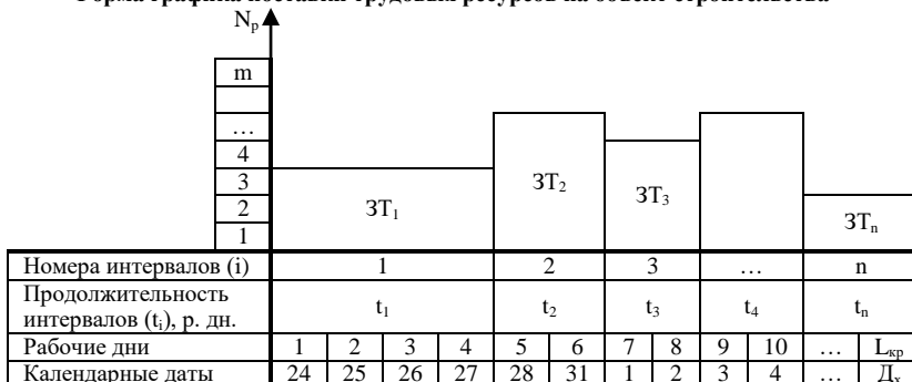
Форма графика поставки трудовых ресурсов на объект строительства
