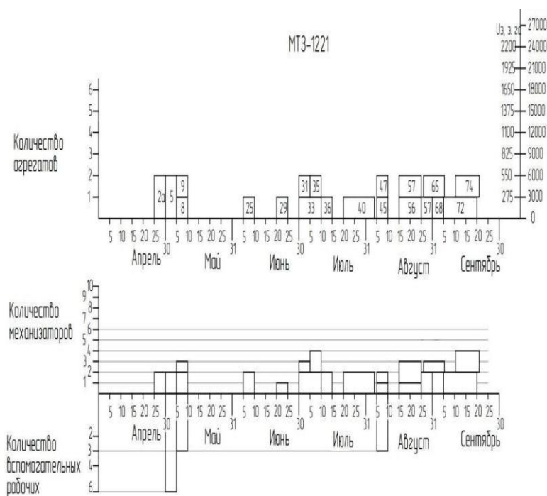
Рис. 2. Графики машиноиспользования и график потребности в трудовых ресурсах (фрагмент)
