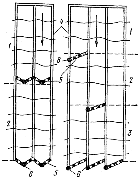
Рис. 28. Размещение стоковых площадок.
