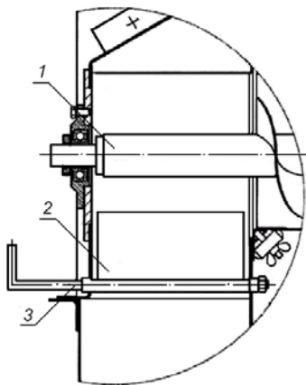
Рис. 10. Распределитель зерна: 1 – шнек; 2 – заслонка; 3 – рукоятка
