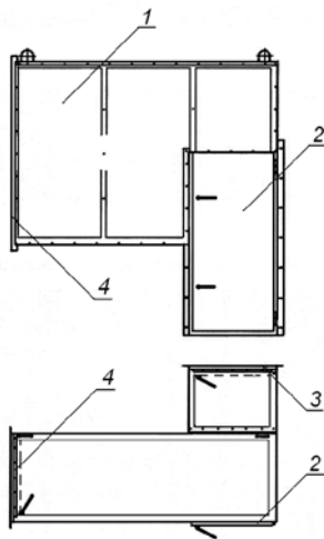
Рис. 11. Воздуховод: 1 – корпус; 2 – наружные двери; 3, 4 – внутренние двери
