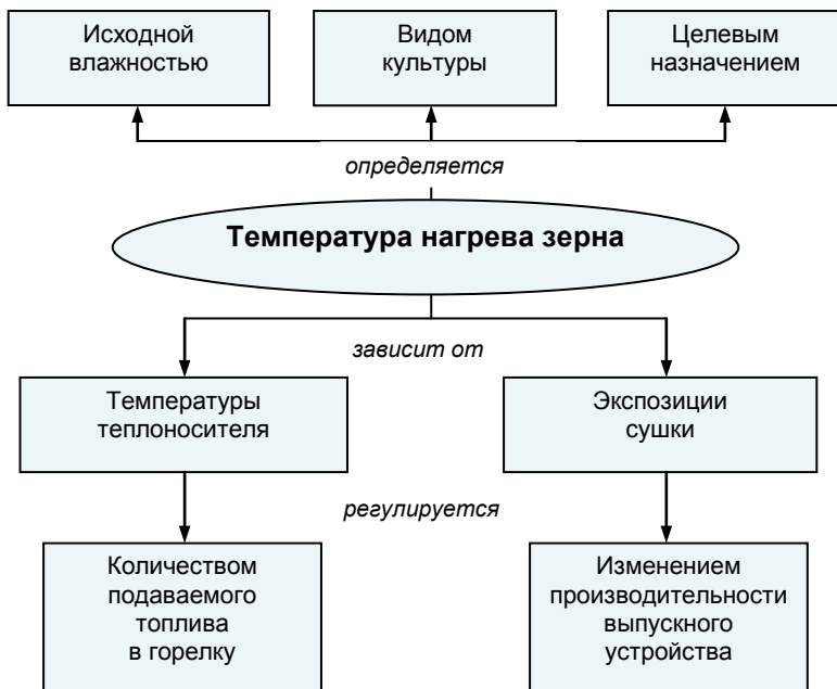
Рис. 6. Структурная схема регулировок зерносушилки М-819
