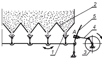
Рис. 5. Выпускное устройство: 1 – лоток; 2 – рассекатель; 3 – эксцентрик; 4 – шатун; 5 – коромысло
