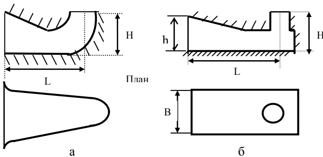
Рис.8.1. Всасывающие трубы: а – криволинейного очертания; б – полигонального очертания
