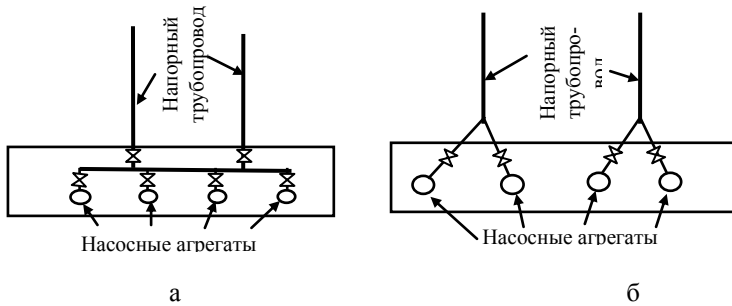
Рис.10.1. Схема переключения напорных трубопроводов: а – полное переключение; б – частичное переключение
