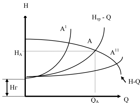
Рис. 3.9. Характеристика трубопровода и рабочая точка
