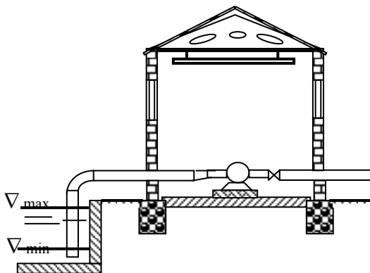
Рис. 11. 5. Схема насосной станции незаглубленного типа.
