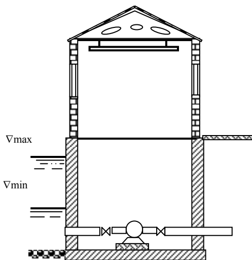
Рис. 11.2. Схема заглубленной насосной станции камерного типа с сухой камерой и насосом с горизонтальным валом.
