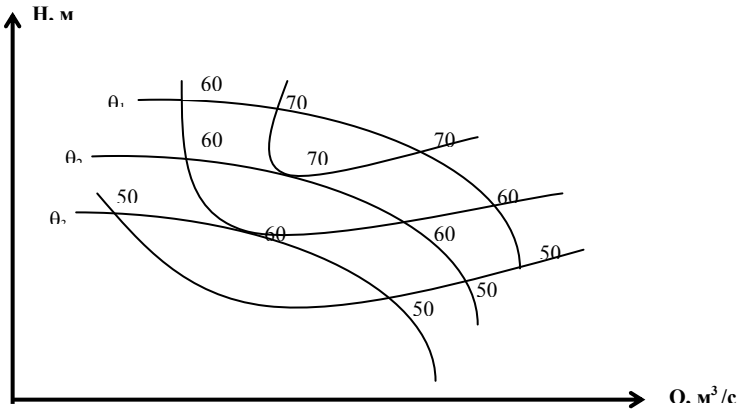
Рис. 3.7. Универсальная безразмерная характеристика осевого насоса
