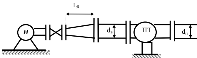
Рис.10.2. Схема внутростанционного напорного трубопровода с переключающим трубопроводом (ПТ)
