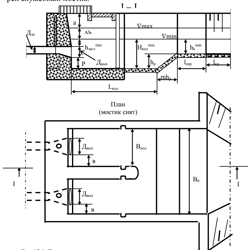
Рис.13.1. Водовыпускное сооружение прямооточного типа с механическим запорным устройством.
