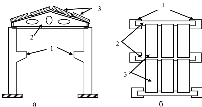
Рис. 11.8. Железобетонный каркас верхнего строения насосной станции: а – разрез; б – план
