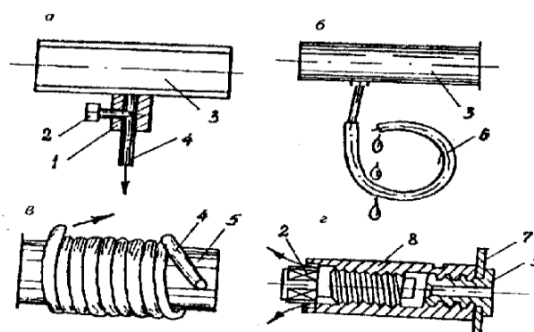
Рис. 7.6. Схема водовыпусков-капельниц; а – микротрубка с винтом для регулирования расходов; б – капельница «Диамонд»; в – капельница «Триклон»; г – капельница типа насадка с винтом; 1 – пробка; 2 – винт; 3 – втулка; 4 – микротрубка; 5 – поливной трубопровод; 6 – трубка-завиток; 7 – стенка поливного трубопровода; 8 – цилиндр
