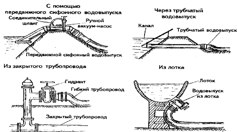
Рис. 7.5. Способы подачи воды в гибкие трубопроводы
