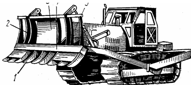
Рис.8.1.Корчеватель-собираатель 1- зубья-клыки; 2- подъемник; 3-основной отвал; 4-балка; 5- уширители
