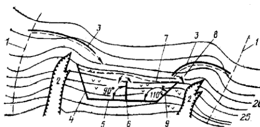
Рис. 8.3. План размещения водозадерживающих валов: 1 – водораздельные линии; 2 – овраги; 3 – водонаправляющие валы-канавы; 4 – глухие шпоры (открытые шпоры); 5 – водозадерживающие валы; 6 – перемычки; 7 – урезы воды; 8 – водообход; 9 – открытая (водосливная) шпора
