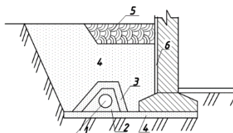
Рис. 5.2. Пристенный дренаж:
