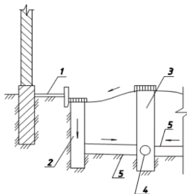
Рис. 5.1. Закрытая ливнесточная система:
