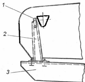
Рис. 4. Схема привода подвижной перегородки: 1 – рычаг; 2 – колебатель; 3 – боковина решетного стана.
