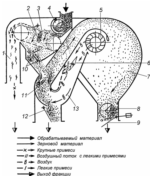
Рис. 1. Схема рабочего процесса машины МПО-50: 1 – выход крупных примесей; 2 – встряхиватель; 3 – сетчатый транспортер; 4 – распределительный шнек; 5 – вентилятор; 6 – заслонка; 7 – отстойная камера; 8 – шнек отходов; 9, 12 – клапаны; 10 – скатные доски; 11, 13 – воздушные каналы.
