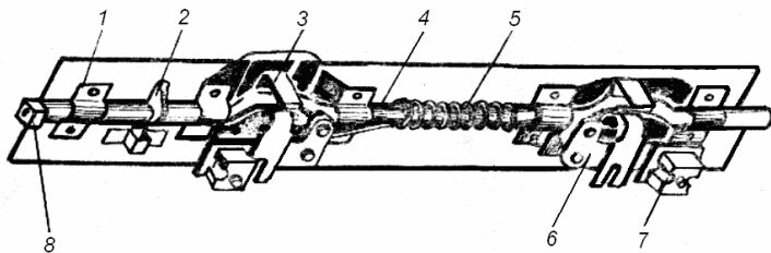
Рис. 5. Механизм зажима щёток: 1 – опора; 2 – кулачок-фиксатор; 3 – кронштейн; 4 – коленчатый вал; 5 – пружина; 6 – рычаг; 7 – ползун; 8 – квадратный конец вала.
