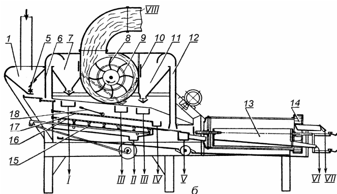
Рис. 10. Схема семяочистительной машины К-531/1: а – общий вид; б – схема работы; 1 – приёмный бункер; 2 – воздушно-очистительная часть; 3 – решётный стан; 5 – питающий валик; 6 – канал первой аспирации; 7, 11 – отстойные камеры; 8 – вентилятор; 9 – сетчатый цилиндр; 10 – заслонка; 12 – канал второй аспирации; 13 – лоток триера; 14 – лопастное (черпаковое) колесо; 15 – щётки; 16 – нижнее решето; 17 – верхнее решето; 18 – колотушка-подбивальщик; I – лёгкие примеси из первой аспирации; II – мелкие примеси; III – лёгкие примеси из второй аспирации; IV – крупные примеси; V – очищенный материал (при работе с выключенными триерами); VI – короткие примеси; VII – очищенный материал; VIII – пыль.
