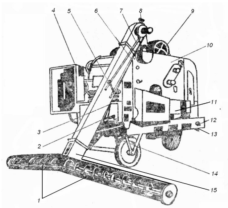
Рис. 2. Семяочистительная машина СМ-4: 1 – питатели; 2 – тяга элеватора; 3 – лебедка; 4 – триеры; 5 – регулировочная гайка; 6, 7 – рукоятки; 8 – натяжники; 9 – отгрузочный элеватор; 10 – воздушно-очистительная часть; 11 – решетный стан; 12 – зерновой шнек; 13 – рама; 14 – механизм самопередвижения; 15 – скребковый элеватор.
