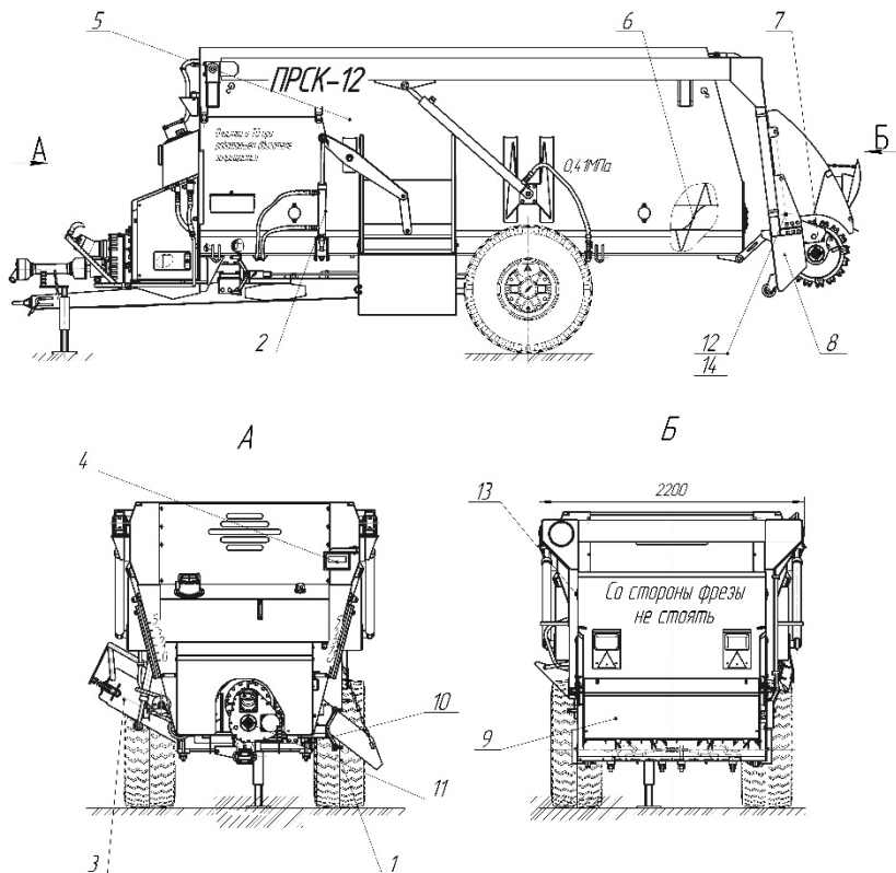
Рис. 1. Погрузчик-раздатчик-смеситель кормов ПРСК-12:
