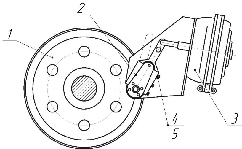
Рис. 11. Тормоз:
