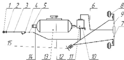
Рис. 6. Тормозная система:
