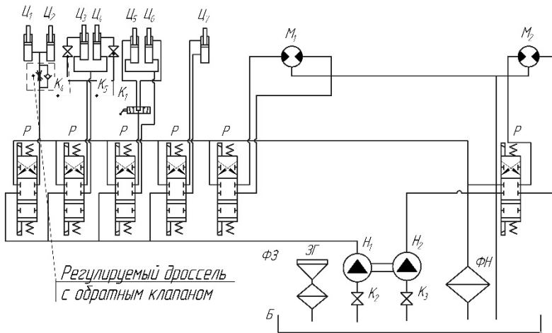
Рис. 5. Принципиальная гидравлическая схема:
