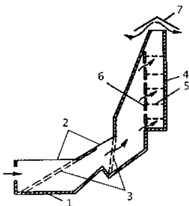
Рис. 15. Солнечная сушилка с пористым абсорбером воздухонагревателя:
