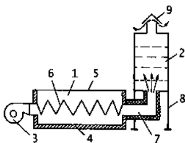
Рис. 14. Солнечная сушилка с вентилятором и гофрированным абсорбером воздухонагревателя:
