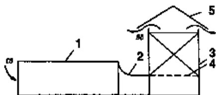
Рис. 13. Камерная сушилка с пленочным воздухонагревателем:
