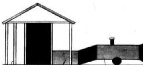
Рис. 19. Сушилка с подогревательной установкой: 1 – каркас с полиэтиленовой пленкой; 2 – стеллажи; 3 – воздуховод; 4 – подогревательная установка.
