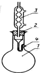
Рис. 14. Прибор для определения содержания эфирного масла методом Гинзбурга: 1 – колба;
