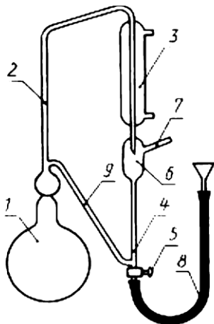
Рис. 15. Прибор для определения содержания эфирного масла методом Клевенджера: 1 – колба; 2 – паропроводная трубка; 3 – холодильник; 4 – градуированный приемник; 5 – спускной кран; 6 – расширение приемника; 7 – боковая трубка приемника; 8 – резиновый шланг; 9 – сливная трубка
