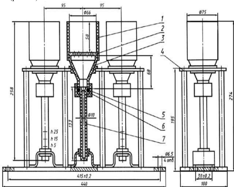
Рис. 20. Устройство типа УЗ-ДУВ для определения водостойкости гранулированных комбикормов: 1 – камера; 2 – сито; 3 – воронка; 4 – корпус в сборе; 5 – прокладка; 6 – гайка; 7 – измерительная трубка
