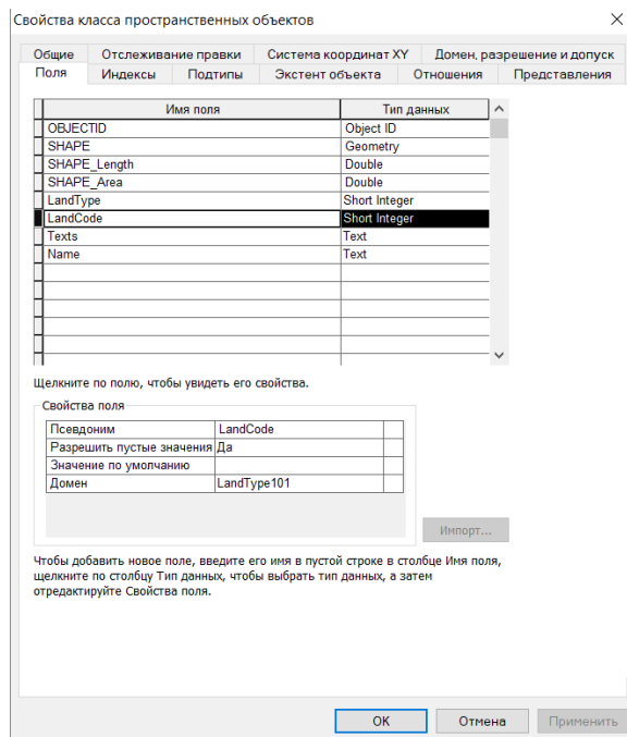
Рис. 18. Установленный домен LandType101 для поля LandCode класса пространственных объектов Land
