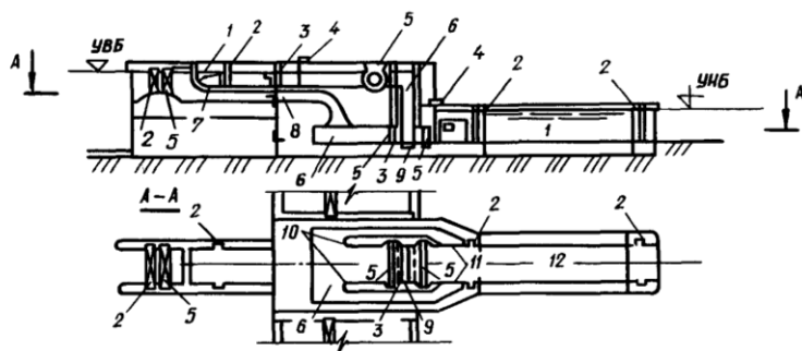
Рис. 1.18. Гидравлический рыбоподъемник:
