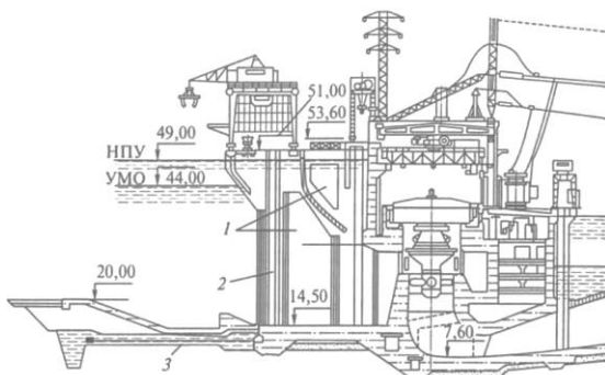
Рис. 1.45. Схемарусловой ГАЭС: 1 – прорези в быках; 2 – пазы в быках; 3 – анкерный понур
