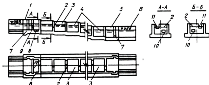
Рис. 1.16. Лестничный рыбоход:
