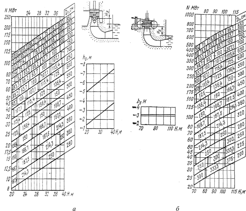
Рис. 1.35. Частные графики применения гидротурбин: а – поворотно-лопастной ПЛ40; б – радиально-осевой РО115
