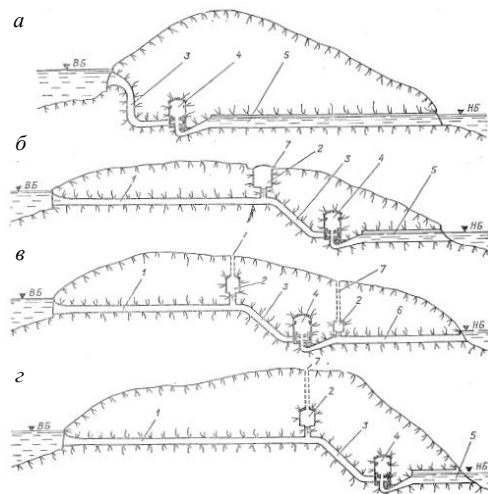
Рис. 1.44. Схема деривационных ГАЭС с подземным размещением машинного зала: а-в – начале туннеля; б и в – в средней части туннеля; г – в конце туннеля; 1 – подводящий напорный туннель; 2 – уравнивающий резервуар; 3 – турбинные водоводы; 4 – машинный зал; 5 – безнапорный отводящий туннель; 6 – напорный отводящий туннель; 7 – воздуховод
