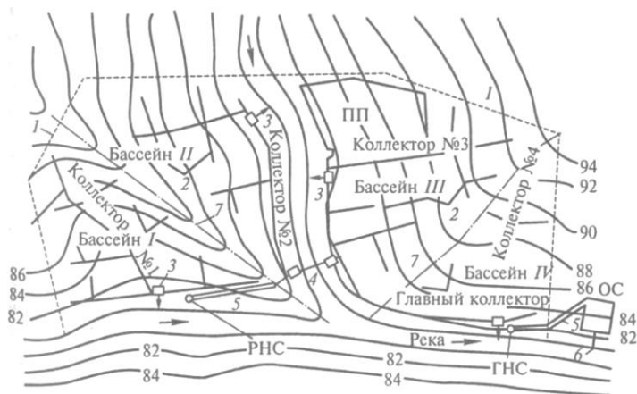
Рис. 1.3. Схема водоотведения: РНС – районная насосная станция; ГНС – главная насосная станция, ОС – очистные сооружения; ПП – промышленное предприятие; 1 – граница города; 2 – внешняя водоотводящая часть трубопровода; 3 – ливнеспуски; 4 – докер; 5 – напорные трубопроводы; 6 – выпуск очищенных сточных вод; 7 – линии водоразделов
