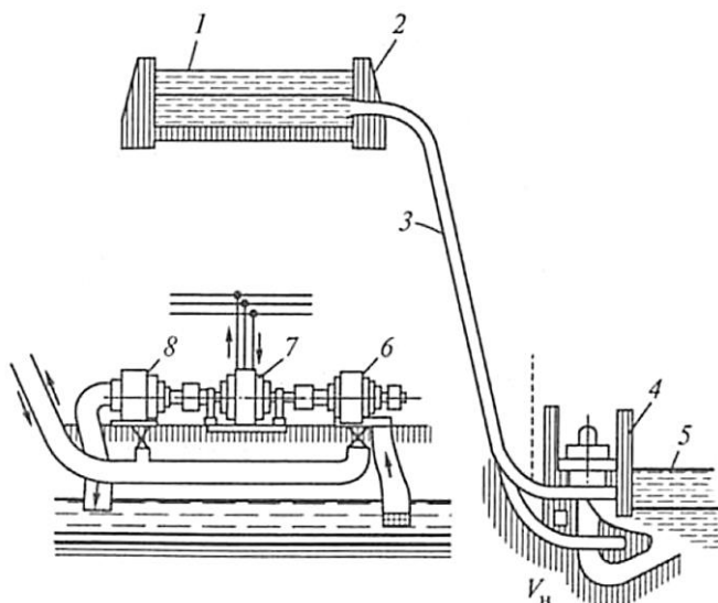
Рис. 1.46. Схема гидроаккумулирующей электростанции: 1 – верхнее водохранилище; 2 – напорный бассейн; 3 – напорный трубопровод; 4 – машинное здание; 5 – нижнее водохранилище; 6 – насос; 7 – двигатель-генератор; 8 – турбина
