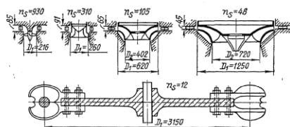
Рис. 1.27. Основные размеры рабочих колес гидротурбин разной быстроходности при N = 1 кВт и H = 1 м (размеры даны в см)
