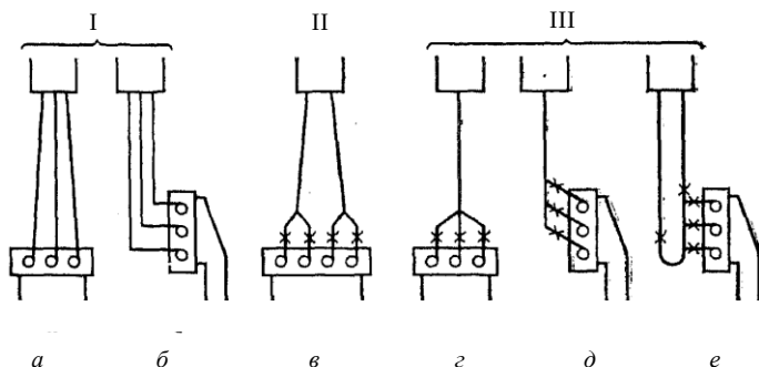
Рис. 1.32. Способы питания турбин при различном подводе трубопроводов к зданию станции: I – раздельное; II – групповое; III – объединенное; а, в, з – фронтальный подвод; б, д, е – продольный подвод
