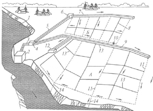
Рис. 1.8. Схема оросительной системы: A – зона самотечного орошения; B – зона машинного орошения; 1 – река; 2 – головное сооружение; 3 – холостая часть магистрального канала; 4 – насосная станина; 5 – напорный трубопровод; 6 – открытый бассейн; 7 – ветвь магистрального канала; 8 – межхозяйственное распределение; 9 – рабочая часть магистрального канала; 10 – дюкер; 11 – водоотводящие каналы; 12 – ГЭС; 13 – внутрихозяйственные распределители; 14 – сбросной канал
