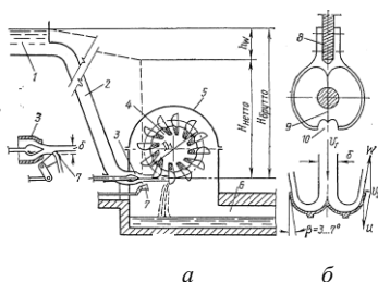
Рис. 1.28. Схема установки с активной (ковшовой) турбиной: а – схема установки; б – схемалопасты (ковша); 1 – напорный бассейн; 2 – турбинный трубопровод; 3 – сопло с регулирующей иглой; 4 – рабочее колесо; 5 – защитный кожух; 6 – отводящий канал; 7 – отклонитель струи; 8 – диск рабочего колеса; 9 – нож ковша; 10 – вырез в ковше для пропуска струи через ковш, находящийся в неблагоприятном положении к струе
