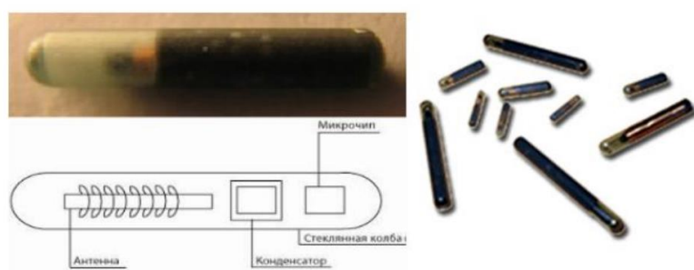
Рис.3. Строение микрочипа
