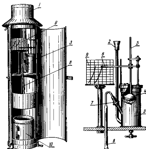
Рис. 4.2. Плювиограф.
