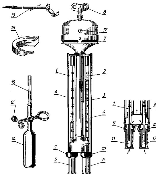
Рис. 3.1. Аспирационный психрометр.
