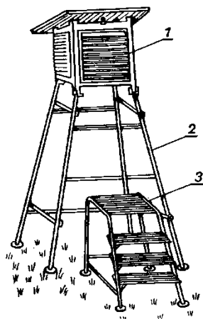
Рис. 2.5. Психрометрическая будка.
