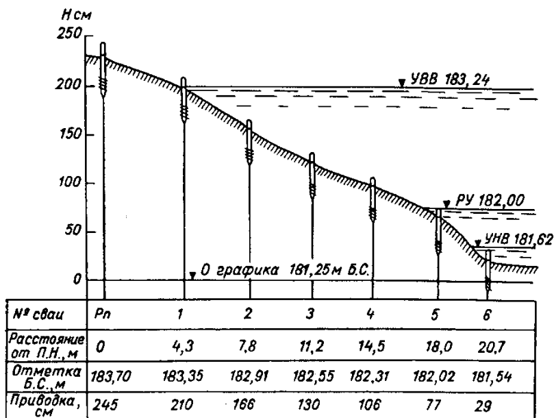
Рис. 7.1. Схема свайного водомерного поста.
