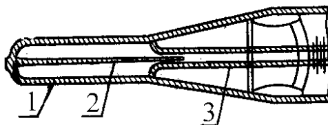
Рис. 2.2. Приспособление для сохранения максимальных показаний термометра.
