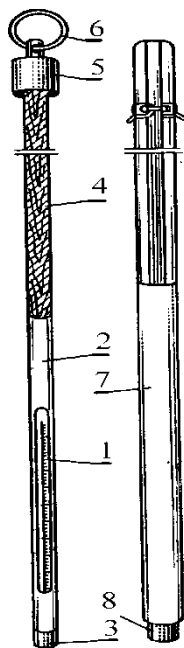
Рис. 2.4. Термометр вытяжной.
