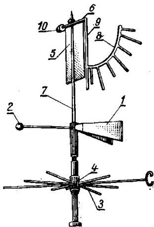
Рис. 6.1. Флюгер.
