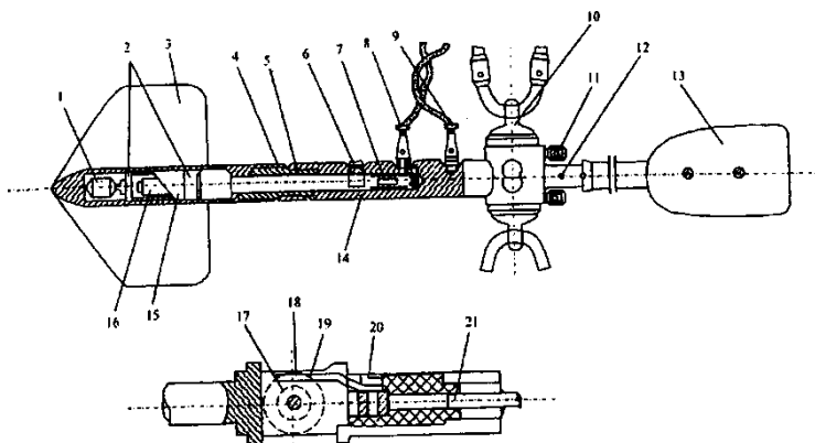
Рис. 9.1. Устройство гидрометрической вертушки ГР-21М: 1 – осевая гайка; 2 – шарикоподшипники; 3 – лопастной винт; 4 – зажимная муфта; 5 – ось; 6 – винт стопорный; 7 – гнездо штепселя; 8 – изолированная клемма; 9 – клемма, соединенная с корпусом; 10 – вертлюг; 11 – зажимные винты; 12 – винт стабилизатора; 13 – стабилизатор; 14 – корпус; 15 – наружная втулка; 16 – внутренняя распорная втулка; 17 – червячная шестерня; 18 – контактный штифт; 19 – контактная пружина; 20 – контактный винт; 21 – токопроводящий стержень.
