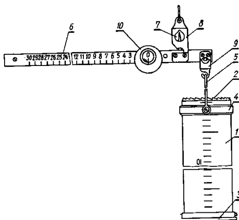
Рис. 4.3. Весовой снегомер.
