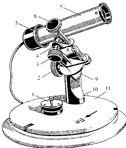
Рис. 1.1. Актинометр термоэлектрический.
