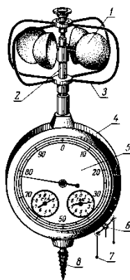
Рис. 6.2. Ручной чашечный анемометр.
