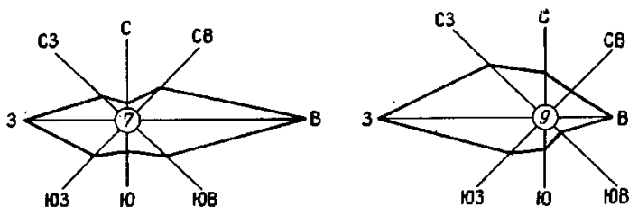
Рис. 6.4. Роза ветров.
