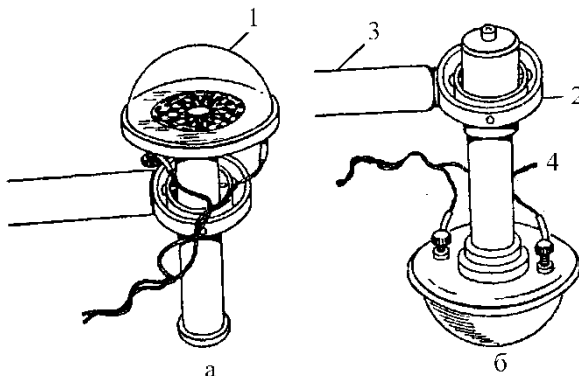
Рис. 1.2. Альбедометр термоэлектрический: а – положение вверх; б – положение вниз.
