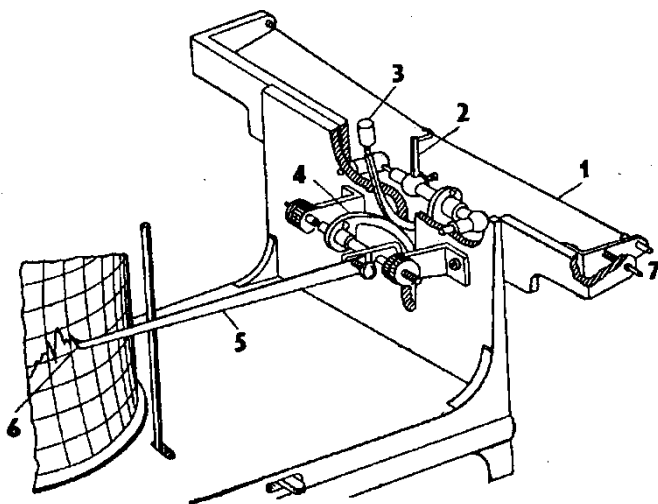
Рис. 3.3. Гигрограф волосной.
