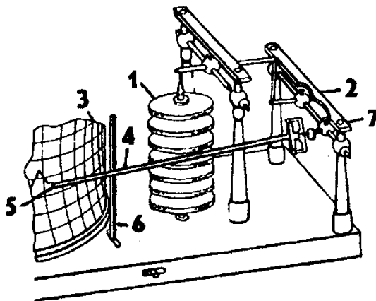
Рис. 5.3. Устройство барографа.
