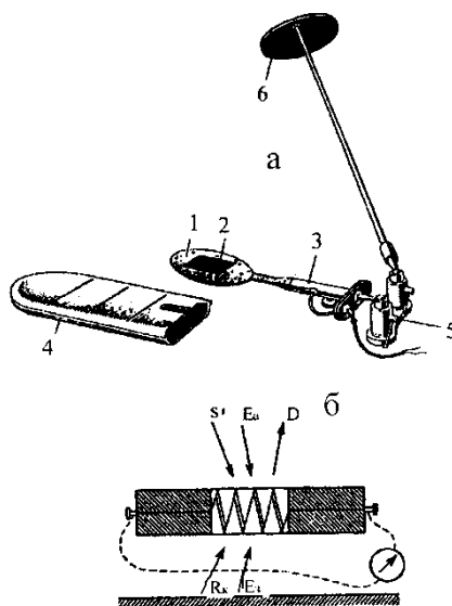
Рис. 1.3. Балансомер термоэлектрический: а – общий вид; б – схема.
