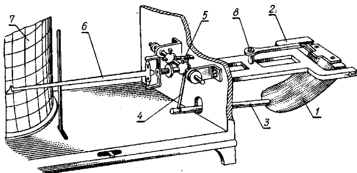
Рис. 2.7. Термограф биметаллический.
