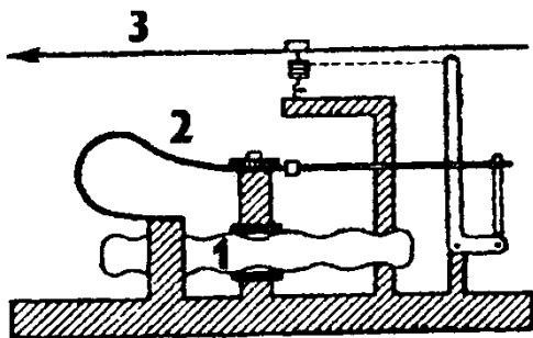
Рис. 5.2. Схема барометра-анероида.
