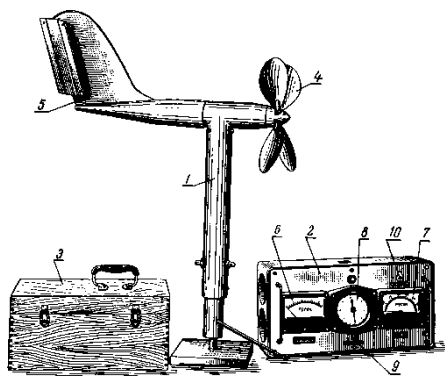
Рис. 6.3. Анеморумбометр.
