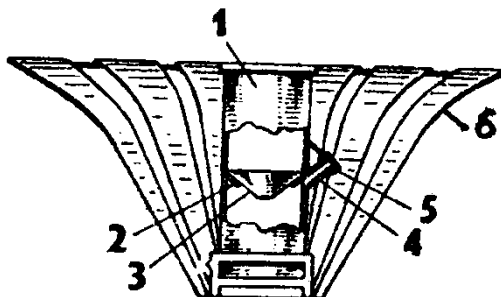
Рис. 4.1. Схема осадкомера Третьякова.
