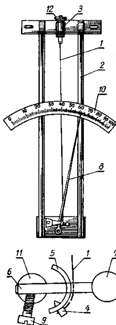
Рис. 3.2. Волосной гигрометр.
