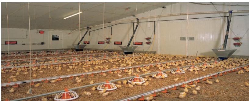
Рис. 40. Напольное содержание цыплят
