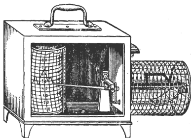
Рис. 7. Термограф
