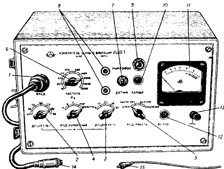
Рис. 25. Прибор для измерения шума и вибрации ИШВ-1
