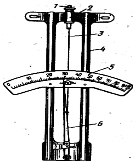
Рис. 12. Гигрометр МВ-18
