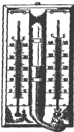
Рис. 10. Статический психрометр Августа
