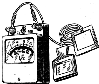
Рис. 18. Люкметр Ю-16
