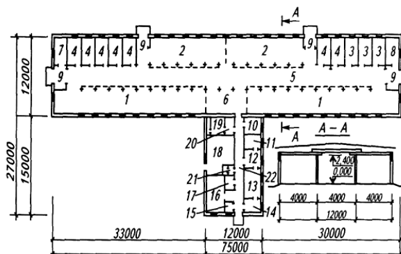
План конюшни на 50 кобыл с кумысным цехом
