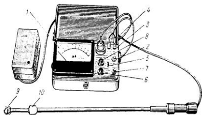
Рис. 6. Термоанемометр ЭА-2М: 1 – гальванометр; 2 – переключатель питания; 3 – клеммы для включения прибора в сеть; 4 – вилка датчика; 5 – переключатель для измерения температуры или скорости воздуха; 6 – переключатель «измерение – контроль»; 7 – ручка регулировки напряжения; 8 – ручка регулировки подогрева; 9 – датчик (микротермо-сопротивление); 10 – защитный футляр датчика
