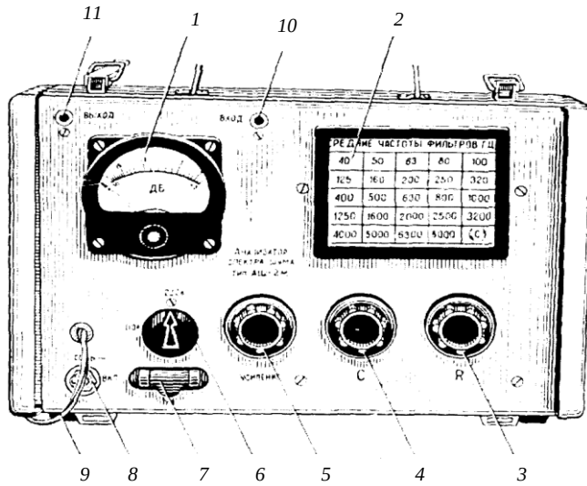
Рис. 24. Анализатор спектра шума АШ-2М
