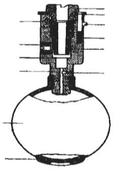
Рис. 20. Универсальный газоанализатор фирмы «Хехст»
