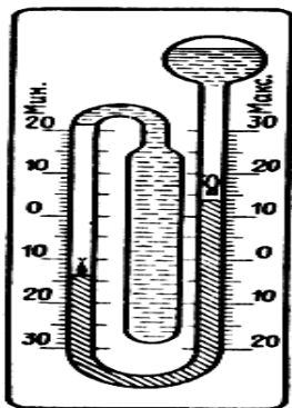
Рис. 5. Максимально-минимальный термометр
