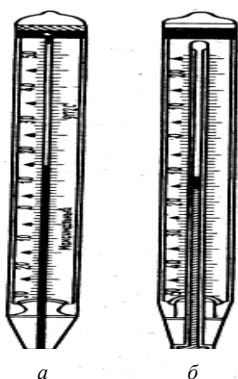
Рис. 4. Максимальный (а) и минимальный (б) термометры
