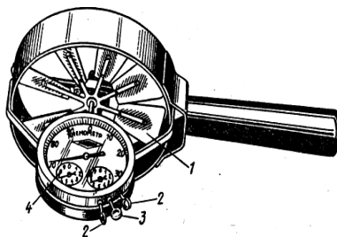
Рис. 16. Анемометр крыльчатый типа АСО-3: 1 – крыльчатка; 2 – ушки; 3 – арретир; 4 – шкала
