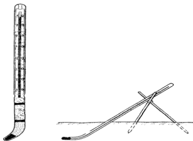
Рис. 26. Почвенный термометр Савинова
