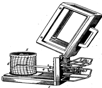
Рис. 13. Гигрограф суточный М-21С
