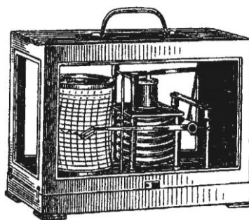
Рис. 9. Барограф М-22С
