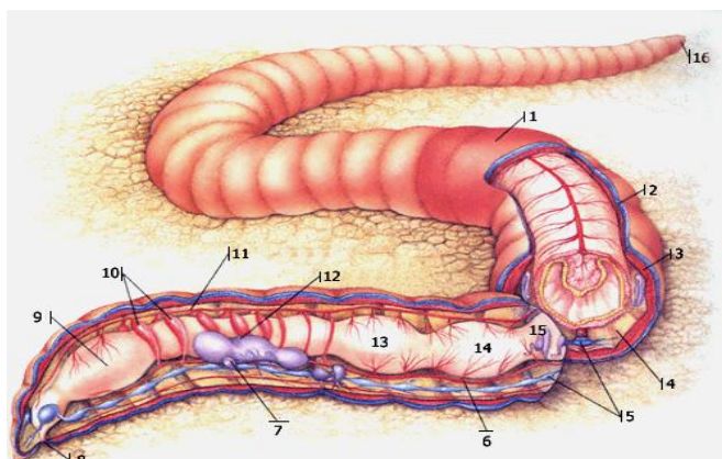
Рис. 21. Дождевой червь:
