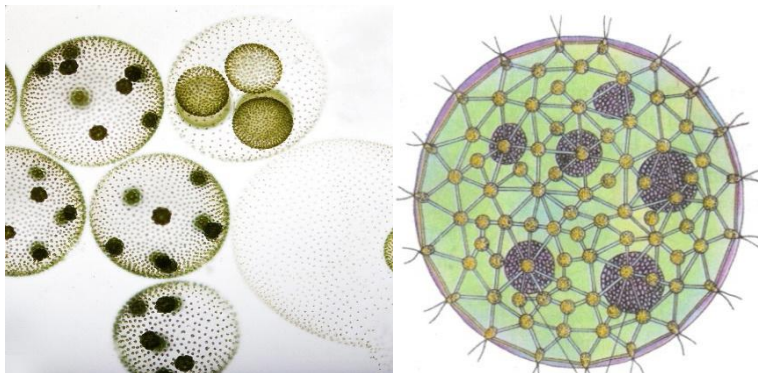
Рис. 4. Вольвокс
