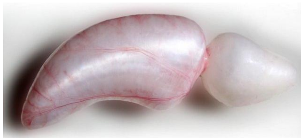
Рис. 55. Плавательный пузырь
