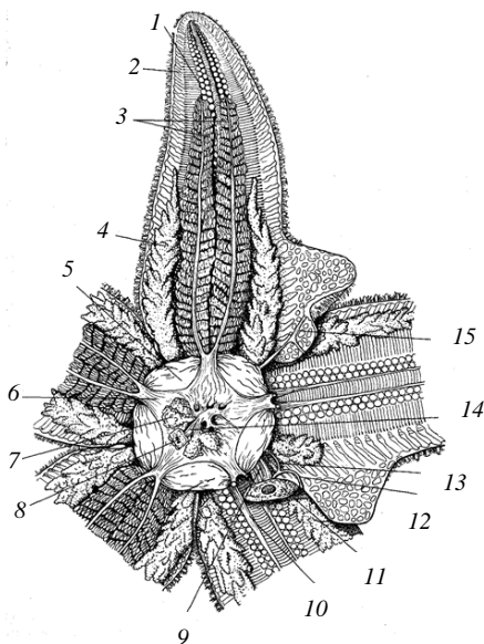
Рис. 31. Морская звезда:
