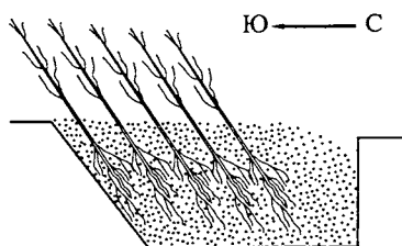
Рис. 4.23. Схема прикопки сеянцев
