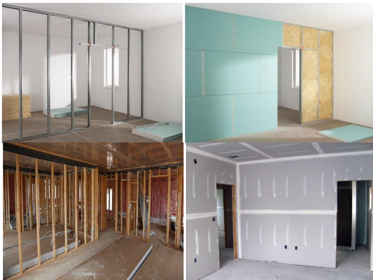
Рис. 28. Перегородки из гипсокартонных листов
