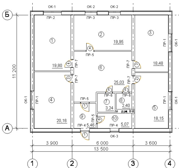
Рис. 81. Обозначение проемов на плане
