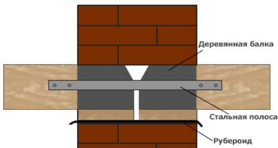
Рис. 64. Опирание деревянных балок на внутреннюю стену
