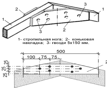
Рис. 142. Коньковая накладка
