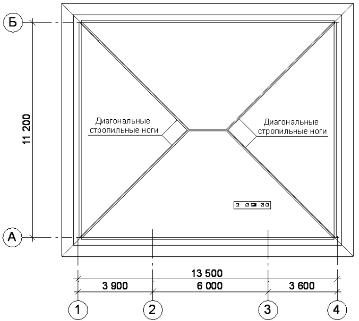
Рис. 150. Расположение диагональных стропильных ног на плане
