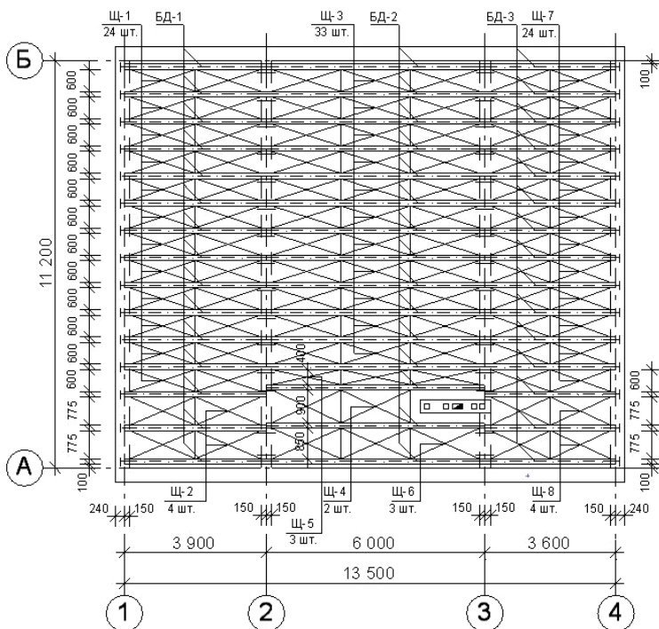
Рис. 175. Пример оформления плана перекрытия по деревянным балкам
