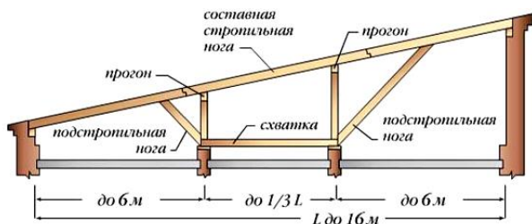
Рис. 92. Стропильная система односкатной крыши (трехпролетные здания)
