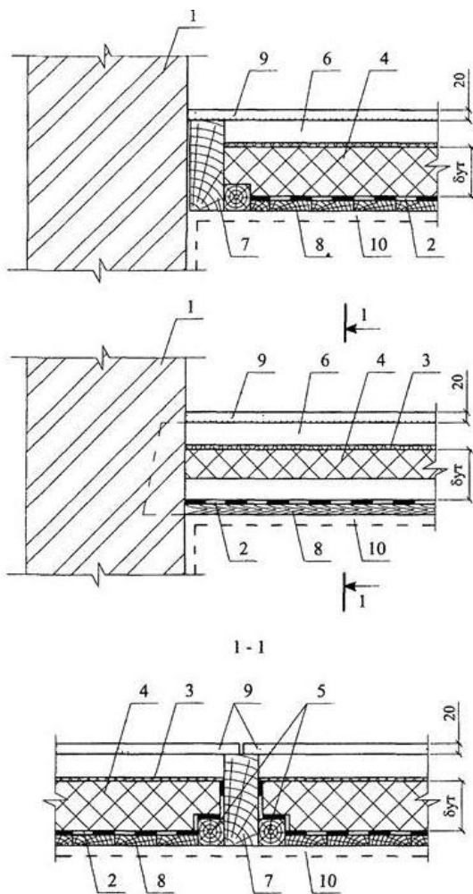
Рис. 66. Элементы чердачного перекрытия по деревянным балкам:
