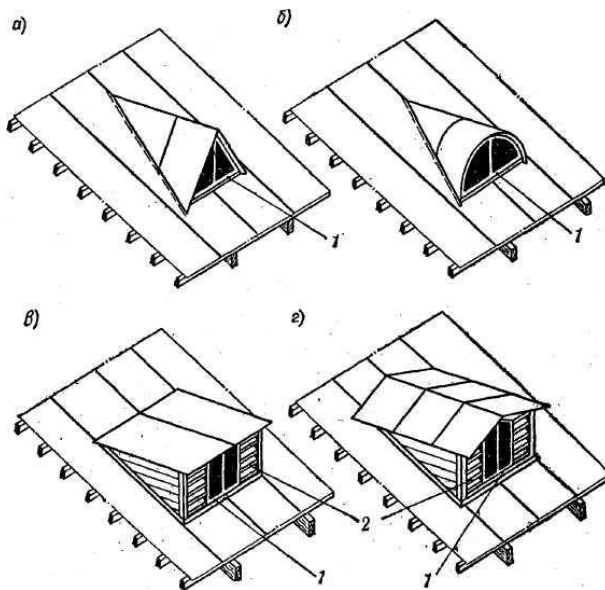
Рис. 127. Формы слуховых окон: а – треугольное; б – полукруглое; в – прямоугольное; г – полигональное; 1 – остекленный переплет; 2 – жалюзийная решетка
