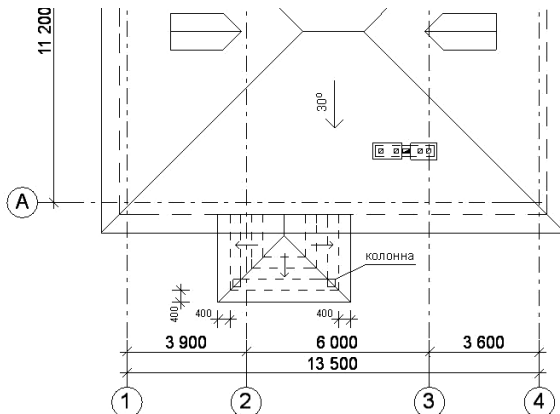
Рис. 164. Крыша над крыльцом с трехсторонним расположением ступеней
