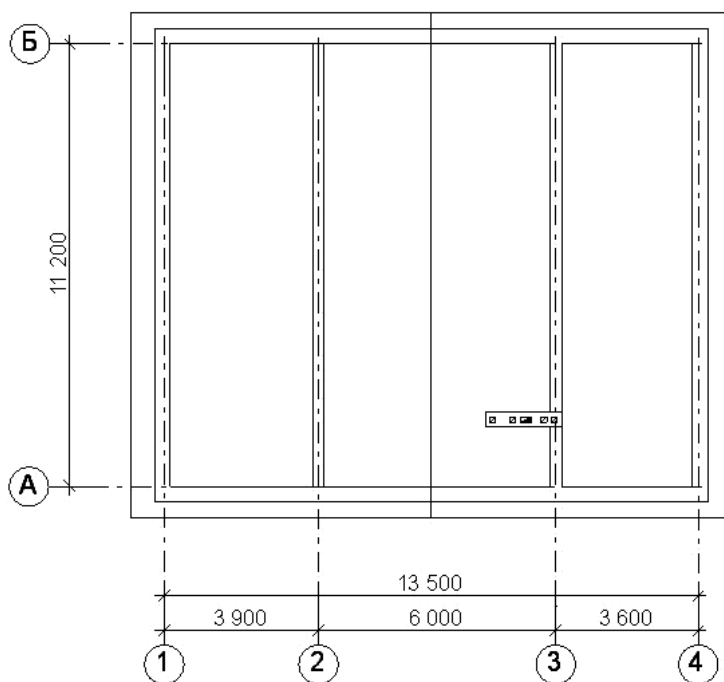
Рис. 139. Наружные и внутренние стены, контур кровли
