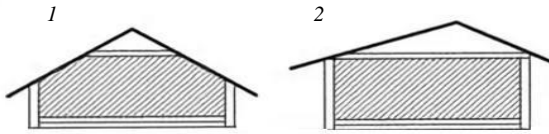
Рис. 132. Варианты устройства двухскатной крыши: 1 – со скатами равной длины; 2 – со скатами разной длины
