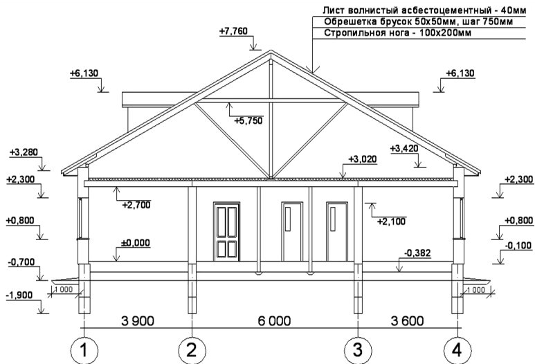
Рис. 188. Разрез 1-1 (двухскатная крыша)
