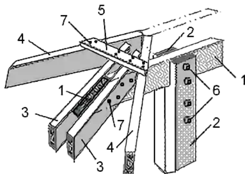
Рис. 152. Опорный узел крепления диагональных стропильных ног на коньковый прогон с опорой на подкосы для вальмового ската: 1 – прогон; 2 – стойка-вилка под прогон; 3 – боковые накладки стропил вальмового ската; 4 – диагональные стропильные ноги; 5 – ригель обрешетки; 6 – болт M12...16; 7 – гвозди
