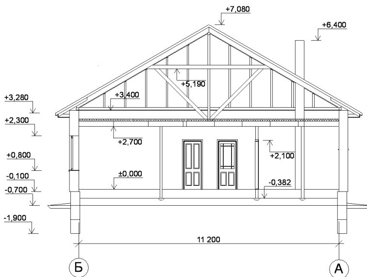
Рис. 189. Разрез 1-1 (вальмовая крыша)
