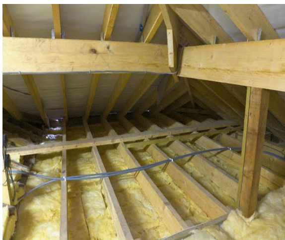
Рис. 49. Пример чердачного перекрытия
