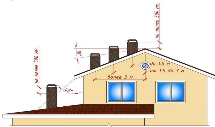
Рис. 21. Расположение трубы над уровнем кровли
