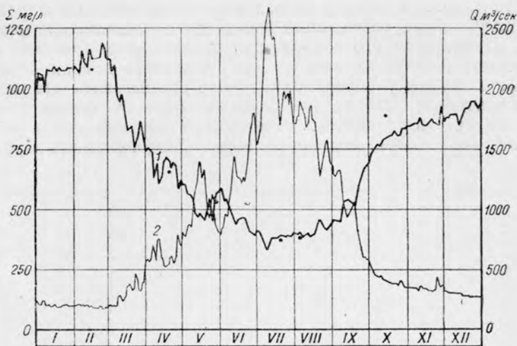
Рис. 33. Изменение минерализации воды ( \Sigma_n ) р. Вахш (кишл. Туткаул) в течение 1942 г. 1 — \Sigma_n , 2 — расход.
