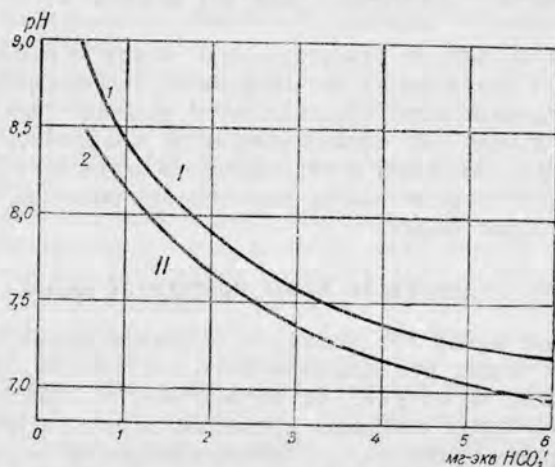
Рис. 10. Изменение величин pH речной воды в зависимости от содержания \text{HCO}_3' и \text{Ca}'' при условии соблюдения произведения растворимости a\text{Ca}'' \cdot a\text{HCO}_3' = 3,6 \cdot 10^{-9} . Кривая II рассчитана для удвоенного количества \text{Ca}'' .
