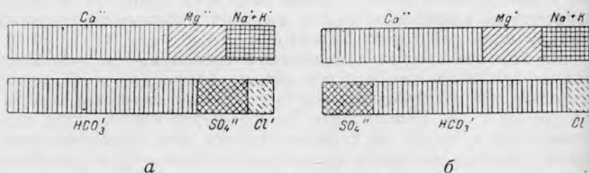
Рис. 21. а) Графическое изображение анализа воды по Роджерсу в видоизменении П. А. Кашинского; б) Видоизмененный график.
