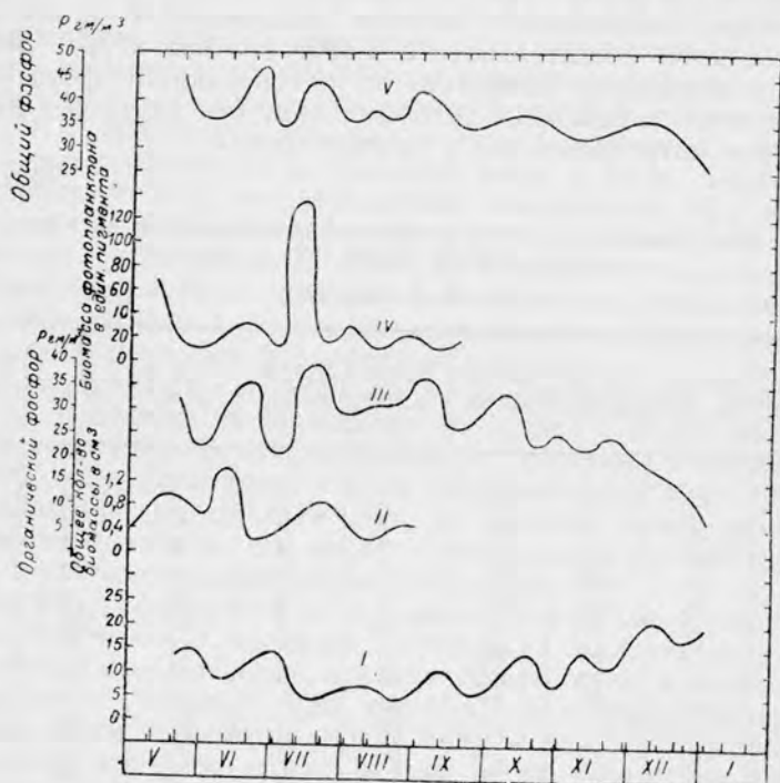
Рис. 58. Распределение неорганического фосфора (I), общего количества биомассы (II), органического фосфора (III), количества фитопланктона (IV) и общего фосфора (V) в слое 5—15 м в районе Вольostrova в Кандалякшском заливе Белого моря (по А. А. Мусиной, П. П. Воронкову и Г. В. Кречману).
