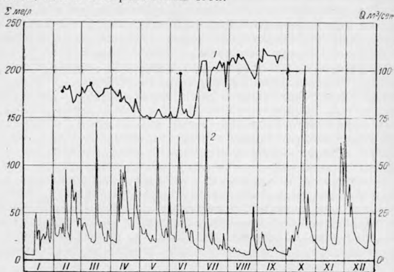
Рис. 31. Изменение минерализации воды (суммы ионов) р. Сочи (ст. Пластунка) в течение 1946 г.
