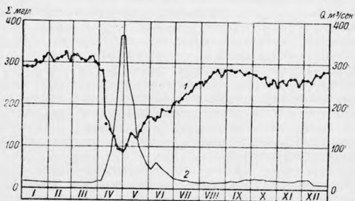
Рис. 32. Изменение минерализации воды ( \Sigma_{и} ) р. Луги (ст. Толмачево) в течение 1946 г.
