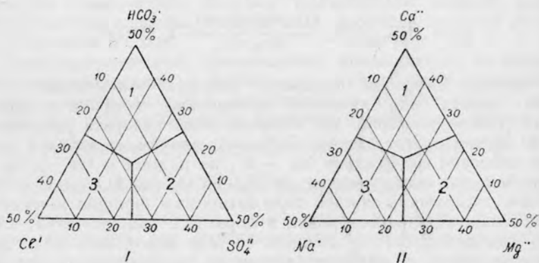
Рис. 18. Треугольная форма диаграмм (анионы и катионы) для обработки результатов большого числа анализов воды.
