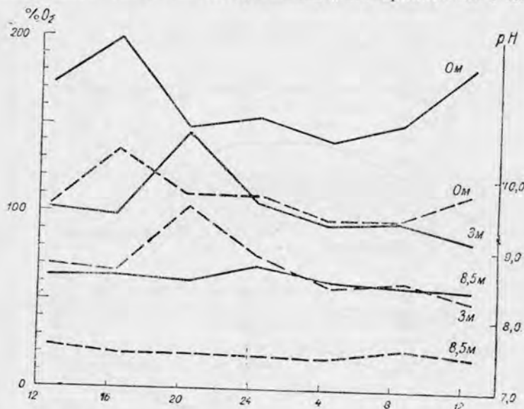
Рис. 52. Суточные изменения насыщения O 2 и pH воды Рыбинского водохранилища 10—11 июля 1947 г. на глубинах 0,3 и 8,5 м (по П. П. Воронкову).
