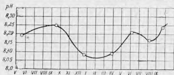
Рис. 60. Сезонное изменение величин pH для глубины 10 м Баренцового моря ( 72^\circ с. ш. и 34^\circ 30' в. д.) (по Е. Крепсу и Н. Вержбинской).
