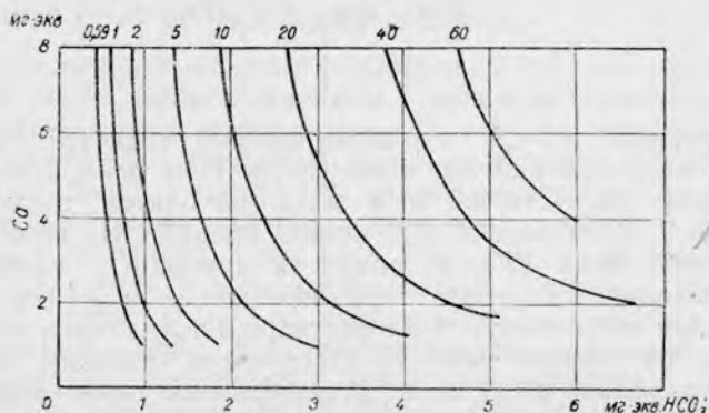
Рис. 13. Соотношение равновесных количеств \text{HCO}_3' , \text{Ca}^{++} и \text{CO}_2 при содержании последней от 0,59 мг/л, т. е. равновесной с атмосферной \text{CO}_2 и до 60 мг/л. Принято, что содержание \text{Mg}^{++} = 0,5 \text{ HCO}_3' (мг-экв); \text{SO}_4^{--} = \text{Ca}^{++} - \text{HCO}_3' ; \text{Na}^+ = \text{Cl}^- и составляют 25% от \text{SO}_4^{--} .
