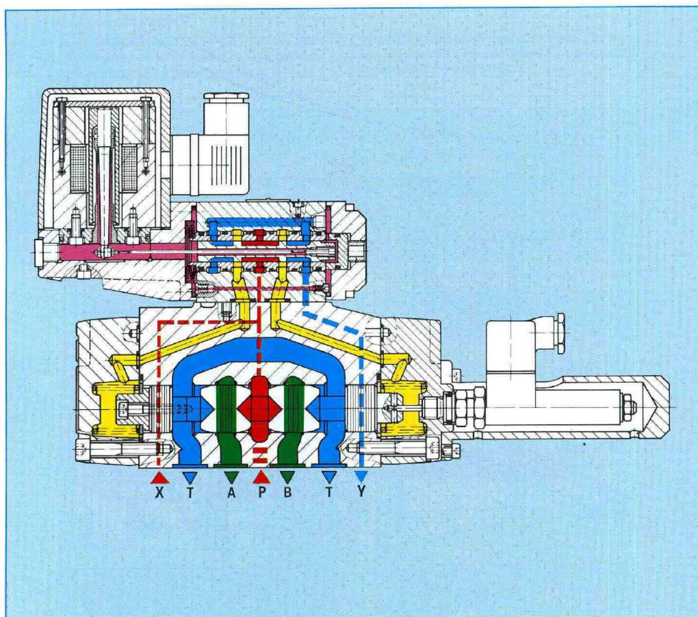
Рис. 30: Пропорциональный распределитель непрямого действия с электрической обратной связью типа 4WRV
