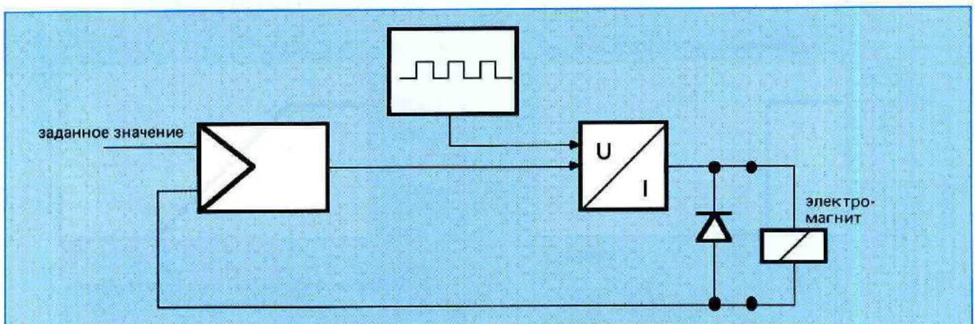
Рис. 4: Импульсно-модулированная конечная ступень
