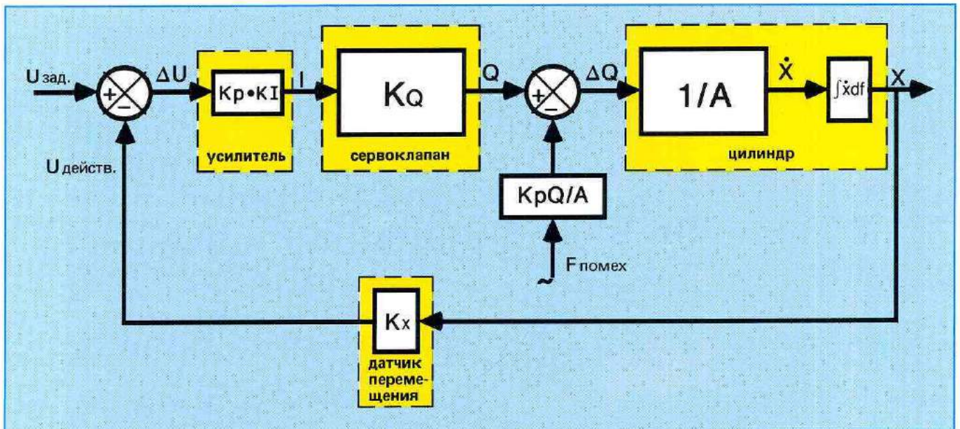
Рис. 2: Упрощенная блок-схема
