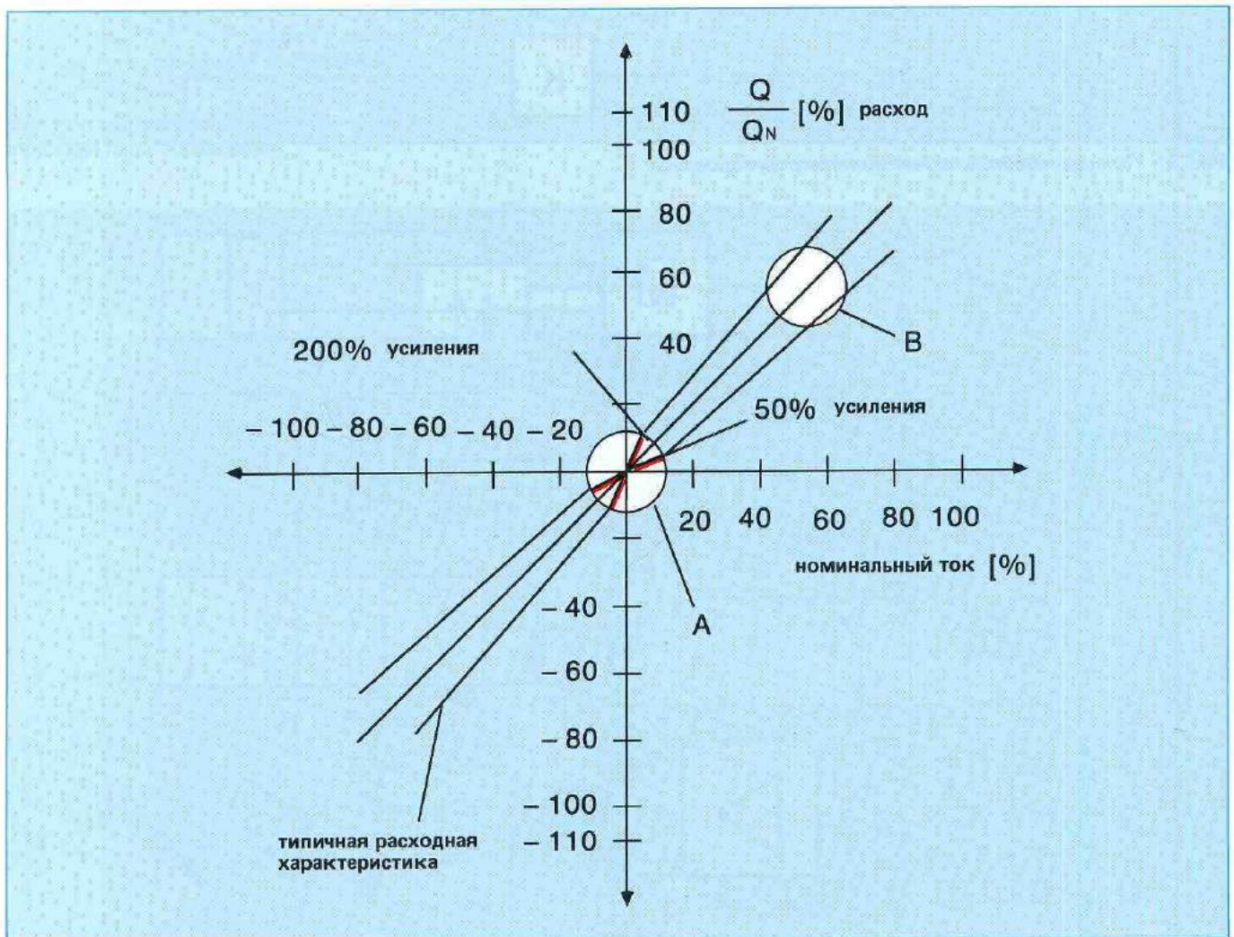
Рис. 5: Расходная характеристика
