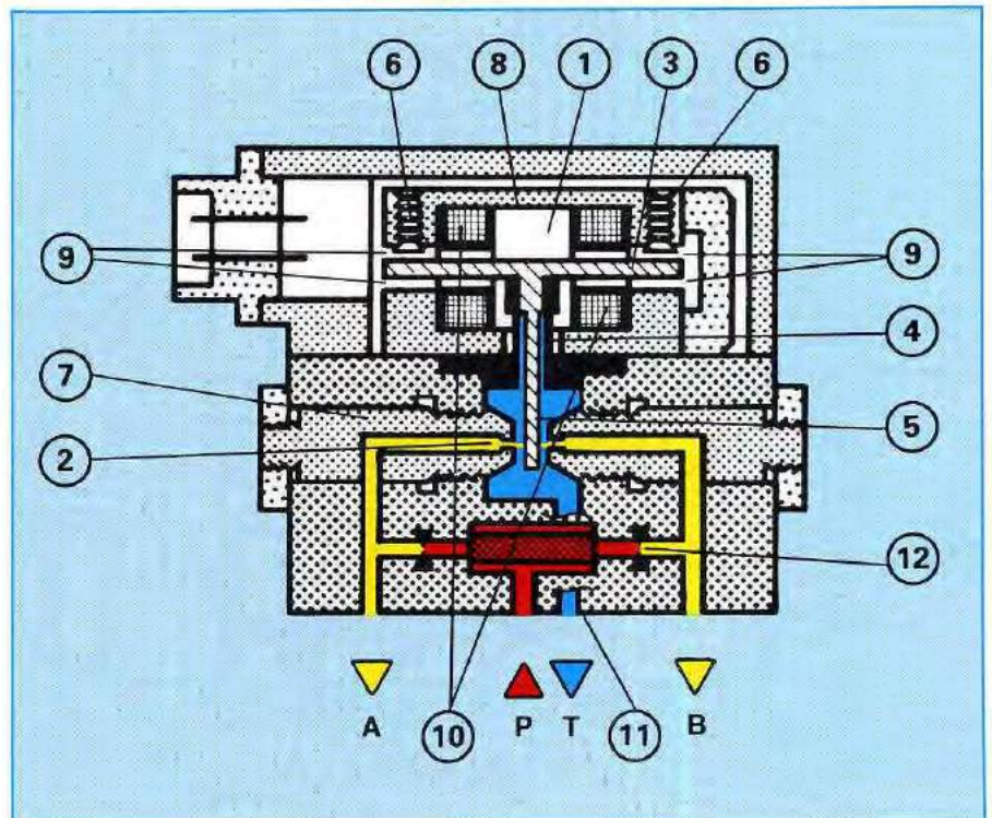
Рис. 8: Принцип системы усиления типа "сопло-заслонка"
