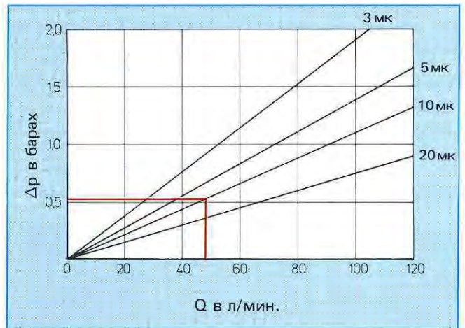
Рис. 15: Диаграмма элемента
