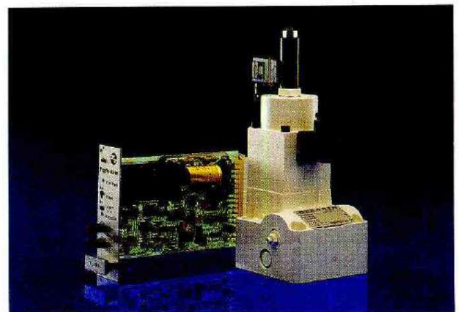
Рис. 56: Двухлинейный пропорциональный регулятор потока типа 2FRE 10, электроника управления
