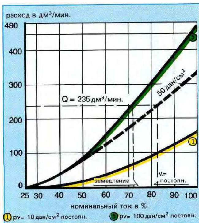
Рис. 17: Графическая характеристика Q - I для номинального расхода в 150 дм 3 /мин. при потере давления клапана в 10 дан/см 2 .
