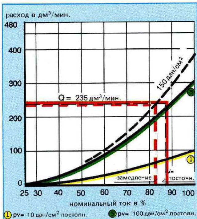
Рис. 14: Графич. характеристика Q - I для номинального расхода в 100 дм³/мин. при потере давл. клап. в 10 дан/см²
