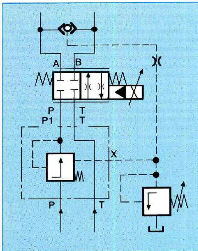
Рис. 15: Впускной клапан постоянной разности давлений с ограничением предельного давления
