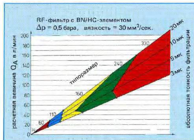
Рис. 17: Диаграмма для определения типоразм. фильтров при фильтрах в сливных линиях с Q до 200 л/мин.
