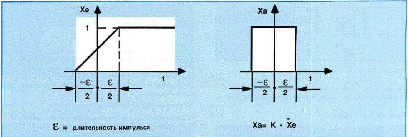
Рис. 22: Переходная характеристика
