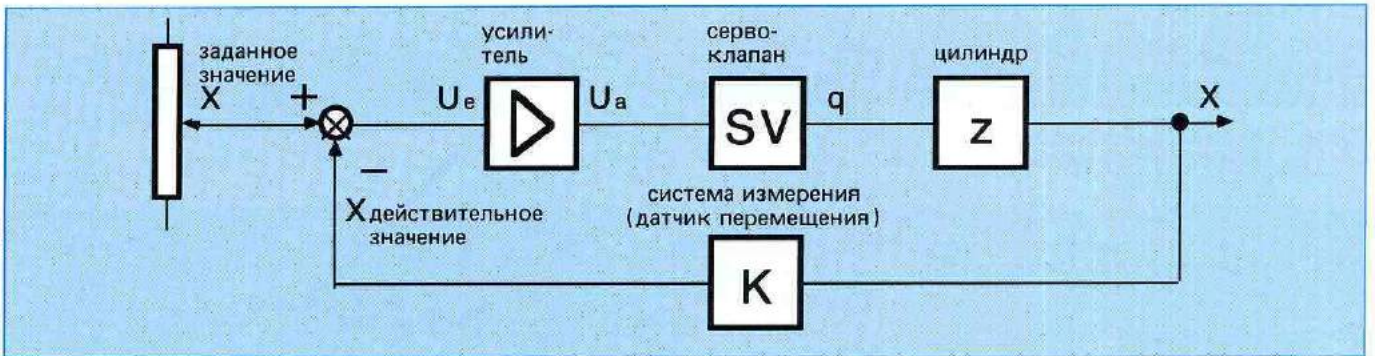
Рис. 3: Упрощенная блок-схема контура регулирования
