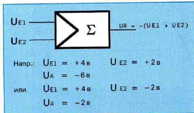
Рис. 11: Сумматор
