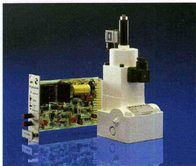
Рис. 7: Пропорциональные регуляторы потока типа 2FRE, электроника управления
