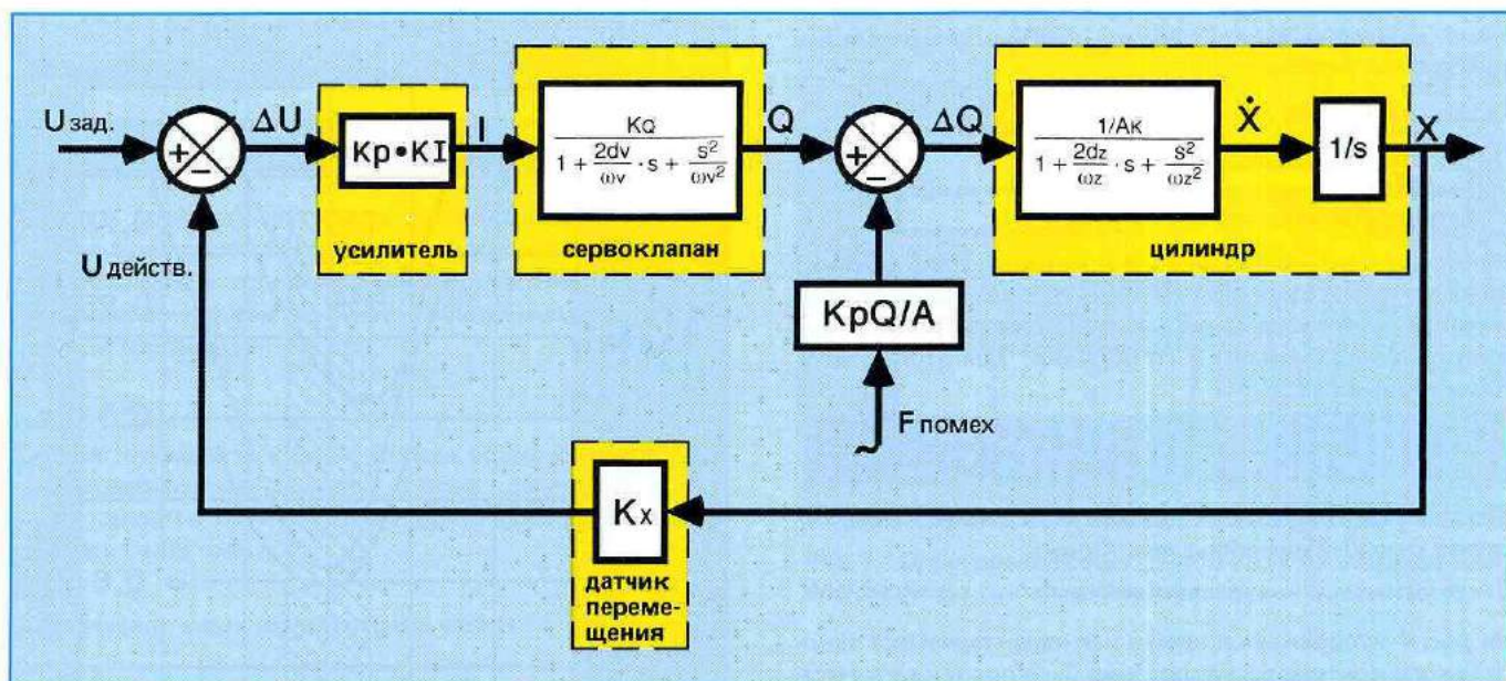
Рис. 3: Подробная блок-схема
