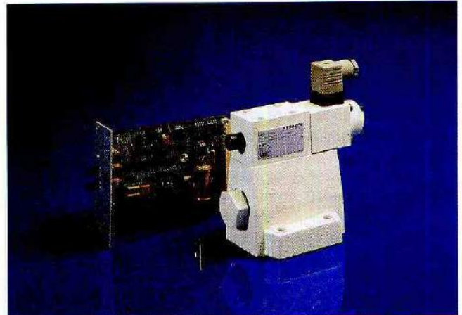
Рис. 46: Пропорциональный редукционный клапан непрямого действия типа DREM 20, электроника управления
