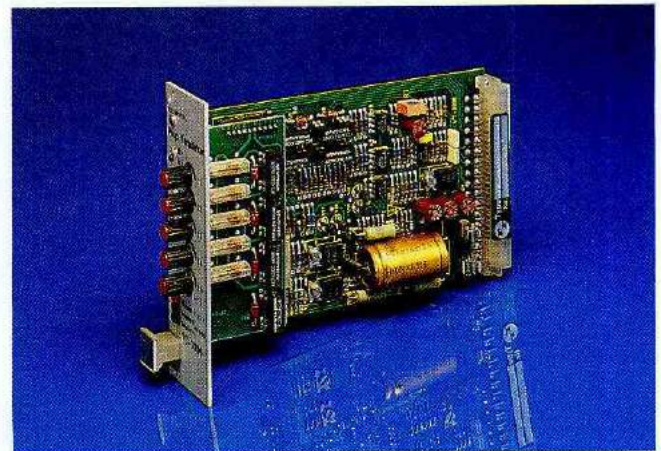
Рис. 21: Линейный усилитель типа VT 3006 S30
