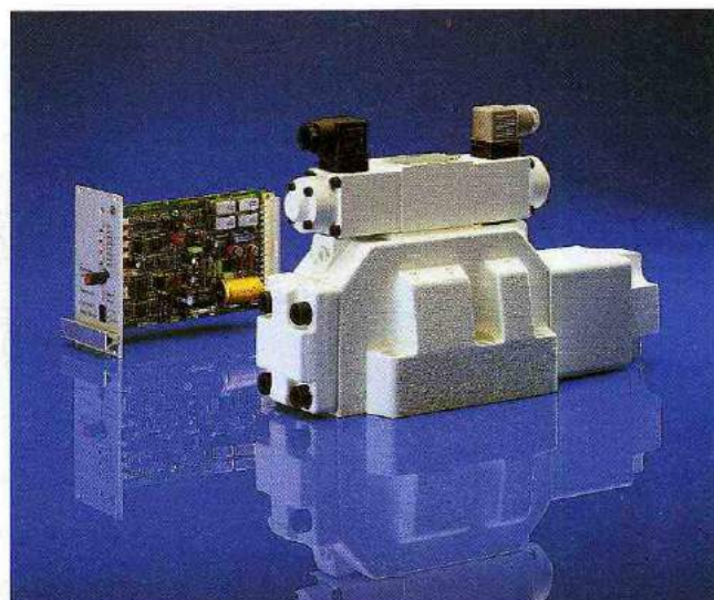
Рис. 5: Пропорциональный распределитель типа 4WRZ, электроника управления
