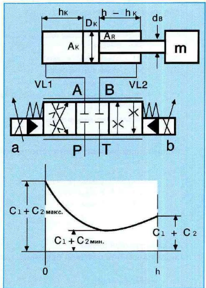
Рис. 25: Дифференциальный цилиндр
