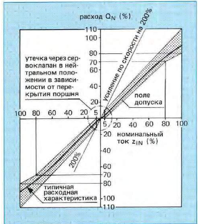
Рис. 13: Поле допуска расходной характеристики сервоклапана
