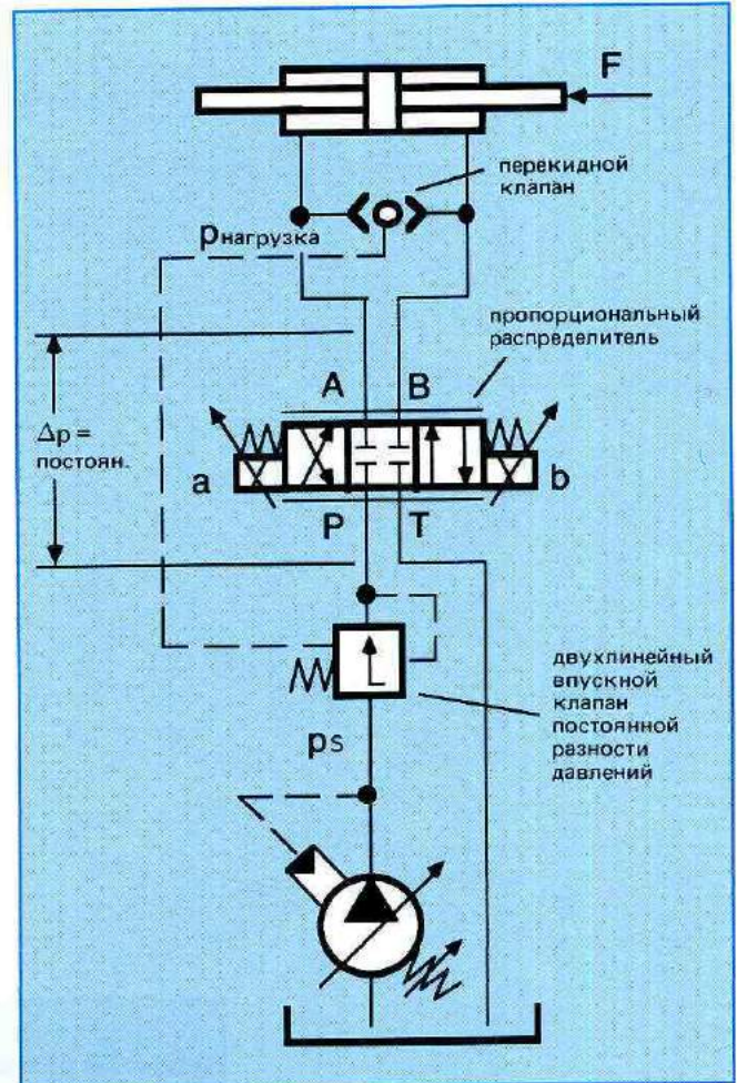
Рис. 2: Пример переключения
