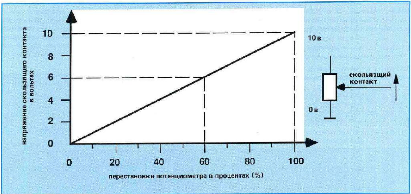
Рис. 84: Потенциометр
