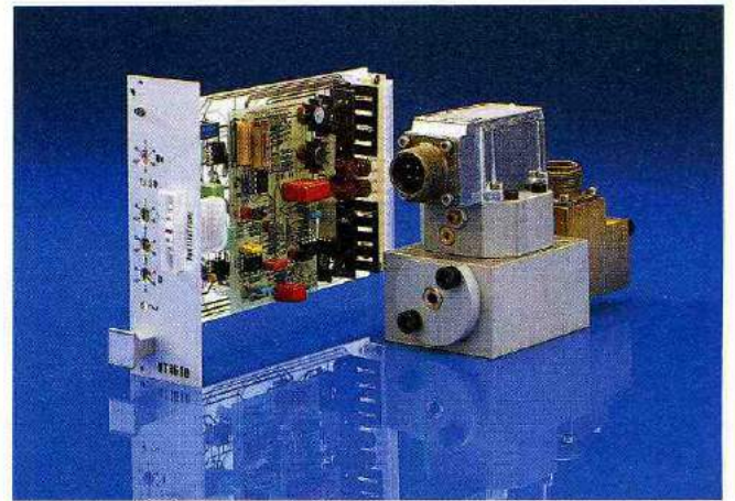
Рис. 20: Двухступенчатый сервораспределитель типа 4WS 2EE 10
