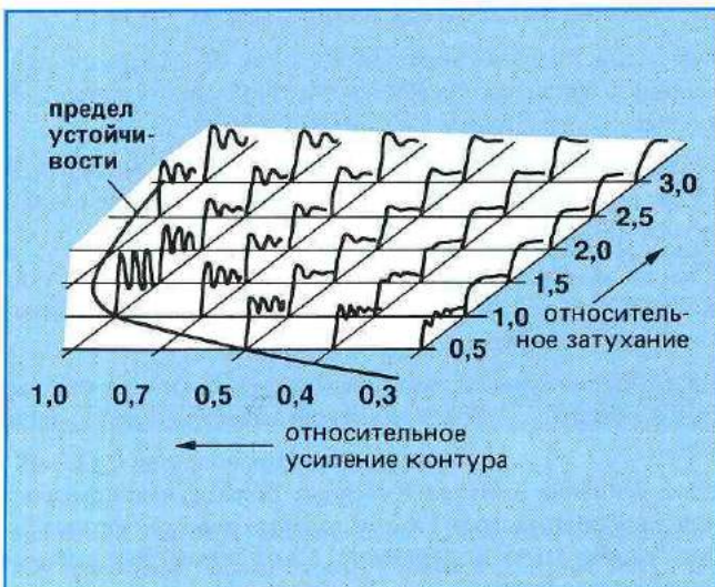
Рис. 4: Временная характеристика контура регулирования 3-го порядка
