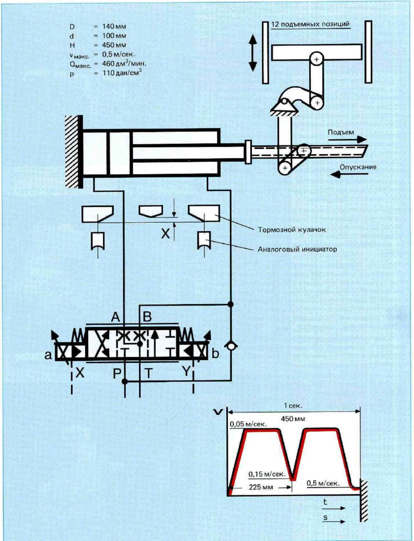
Рис. 4: Принципиальная схема гидромеханического привода на поточной линии сварки (наверху) и его ход перемещений на диаграмме (справа внизу).
