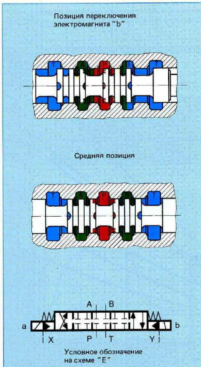
Рис. 11: Перекрытие переключающего распределителя ДУ25, условное обозначение на схеме "E" (закрытая средняя позиция)
