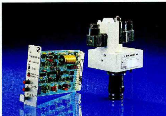
Рис. 57: Двухлинейный пропорциональный дроссель типа FE..C, электроника управления
