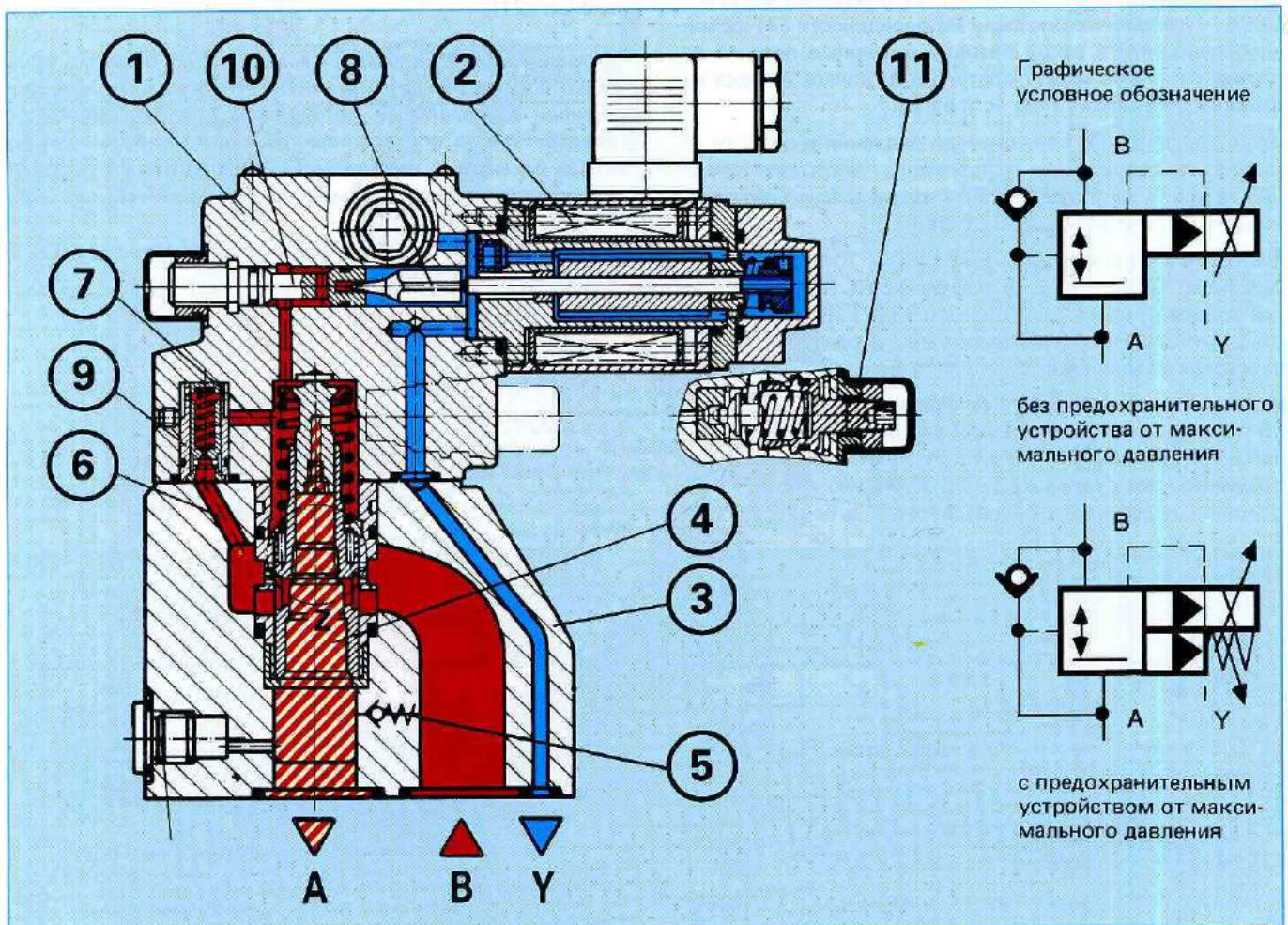
Рис. 49: Пропорциональный редукционный клапан непрямого действия типа DRE 30/DREM 30
