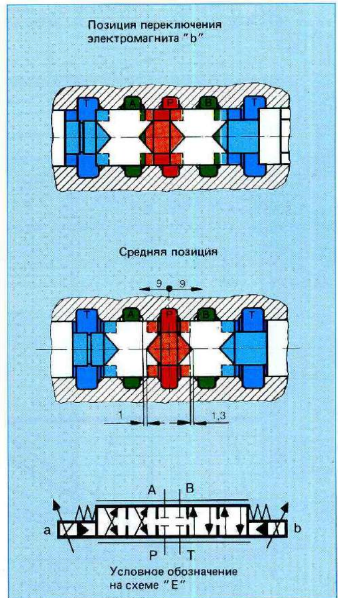
Рис. 12: Перекрытие пропорционального распределителя ДУ25, условное обозначение на схеме "E" (закрытая средняя позиция)
