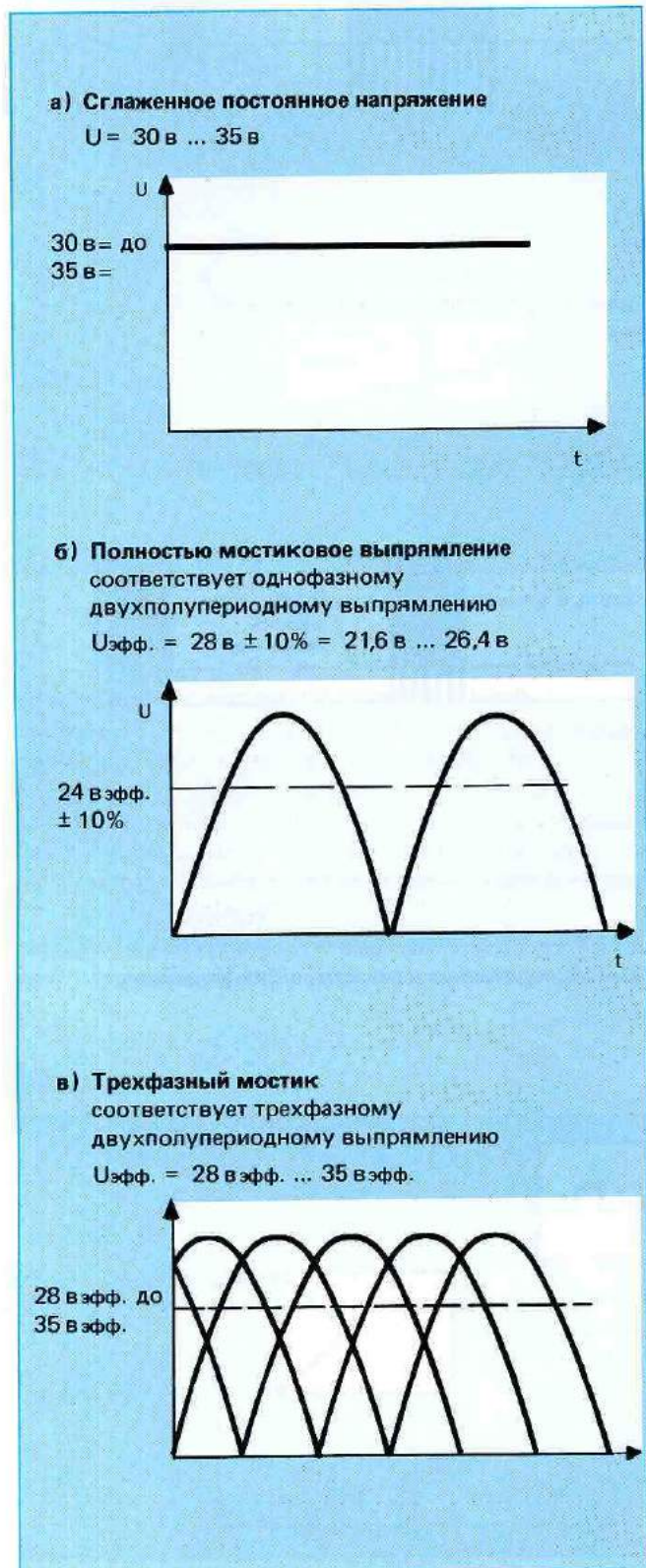
Рис. 6: Питание напряжением
