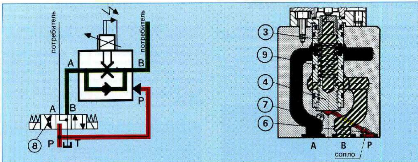
Рис. 52: Внешнее заперение клапана постоянной разности давлений
