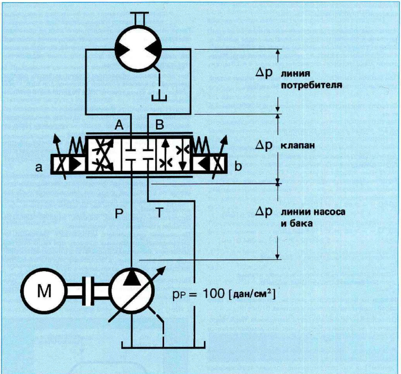
Рис. 21: Потеря давления в одной гидросистеме
