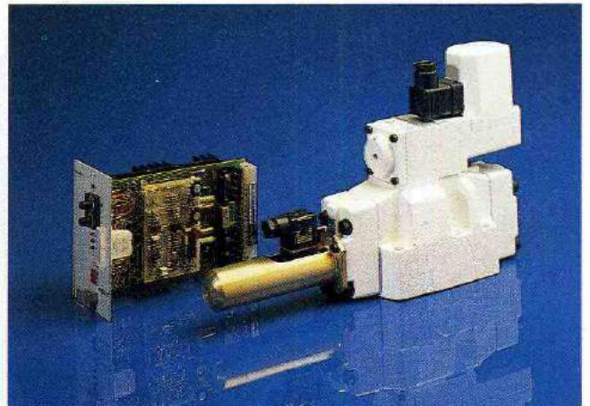
Рис. 4: Двухступенчатый пропорциональный распределитель типа 4WRV, в качестве 1-й ступени применяется регулирующий клапан (рис. 3)
