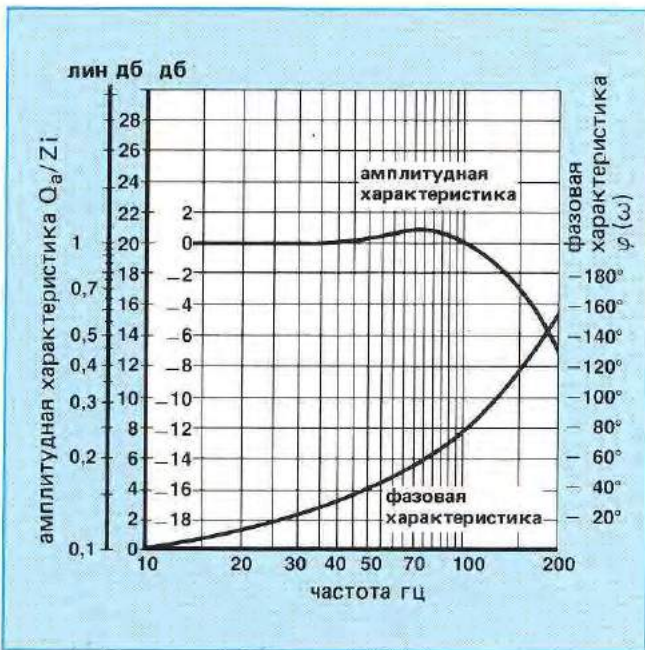
Рис. 13: Диаграмма Боде
