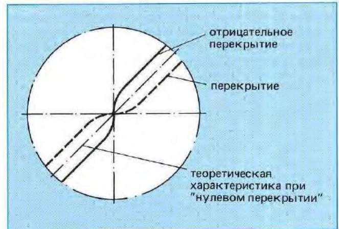
Рис. 14: Принцип перекрытия поршня
