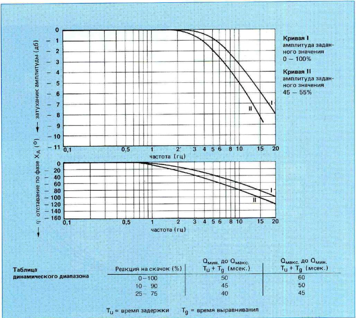
Рис. 55: Частотная характеристика
