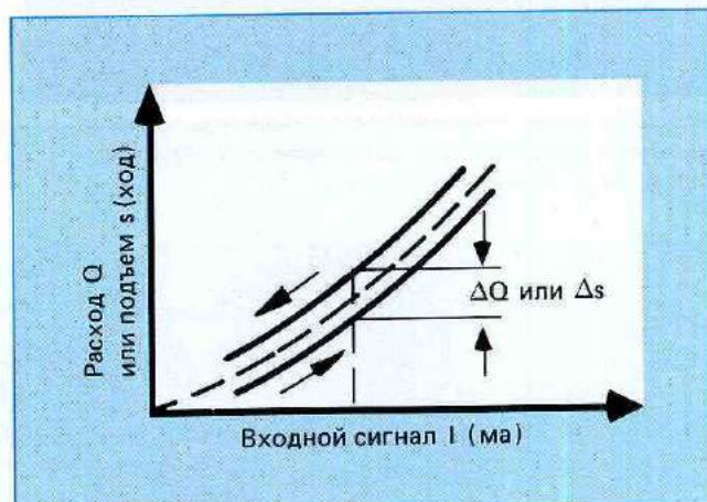
Рис. 8: Гистерезис
