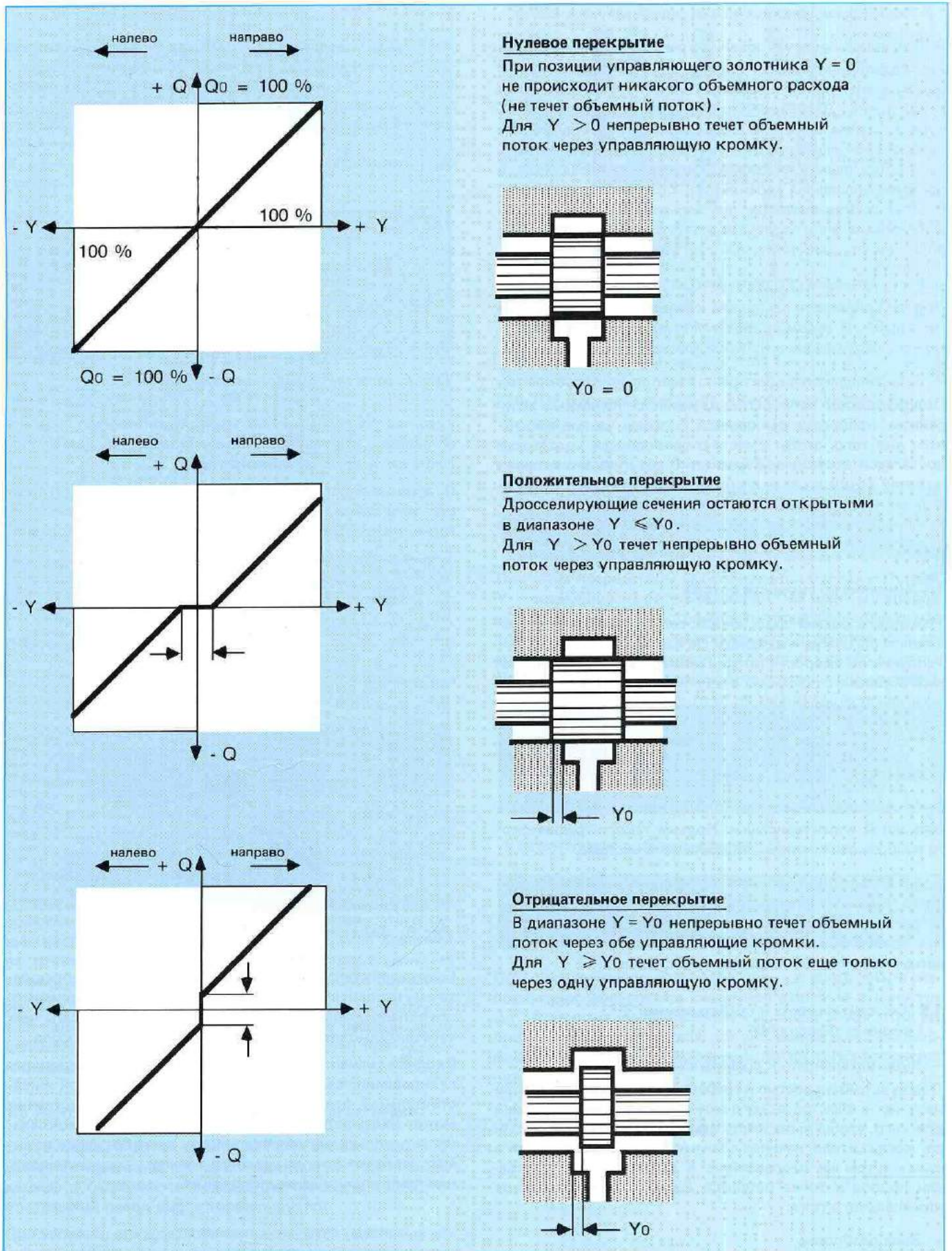
Рис. 6: Расходная характеристика для отличающихся перекрытий в нулевой точке (точка A)
