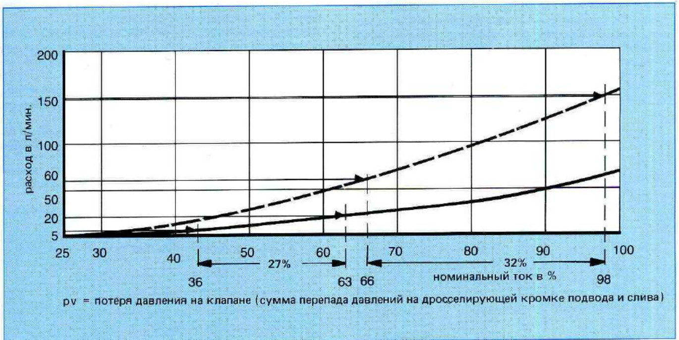
Рис. 14: Характеристика "расход - номинальный ток" для номинального расхода в 64 л/мин. при потери давления на клапане в 10 бар.
