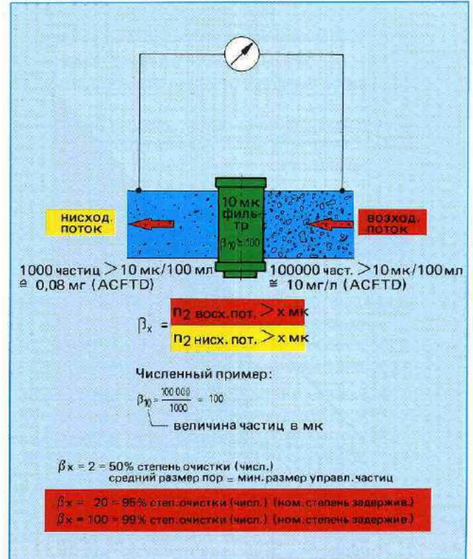
Рис. 9: Изображение отделения частиц загрязнения посредством фильтроэлементов
