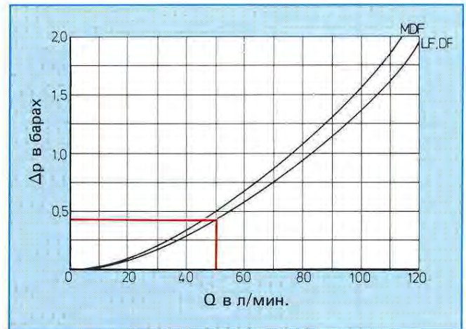
Рис. 14: Диаграмма корпуса из проспекта напор. фильтра
