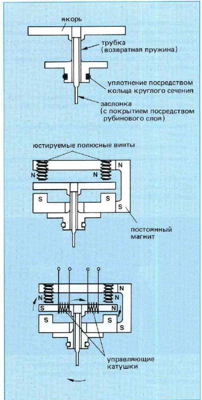
Рис. 5: Конструкция серводвигателя
