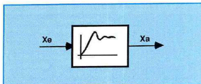
Рис. 32: Символ для P-T 2 -звена
