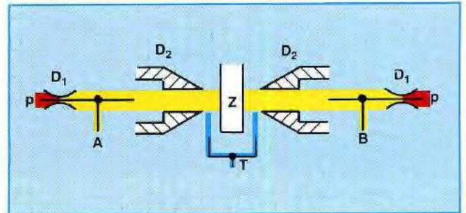
Рис. 8: Принцип системы усиления типа "сопло-заслонка"
