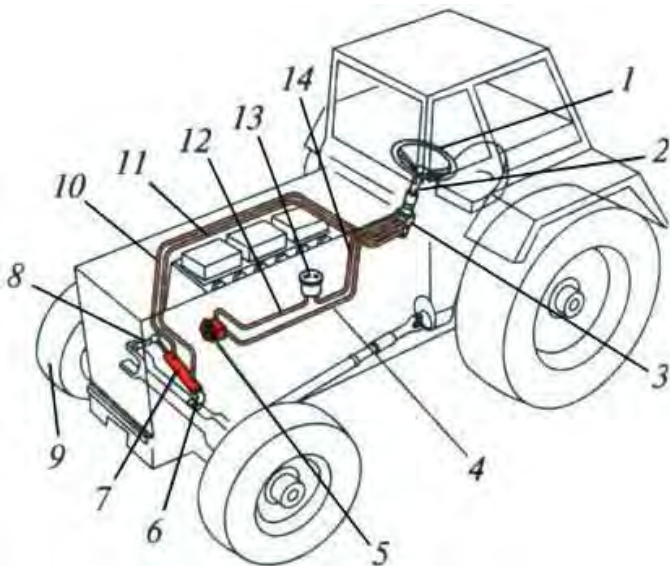
Рис. 2. Одноконтурное ГОРУ: a – схема; б – компоновка на тракторе.
