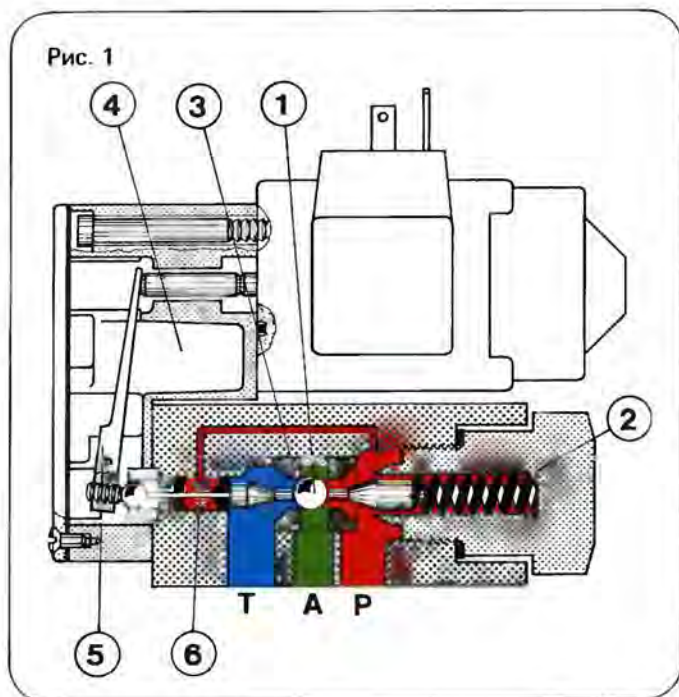
3/2-ходовой седельный клапан с одним шаровым затвором, тип SE..U
