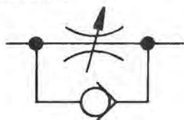
Дроссельный обратный клапан тип МК
