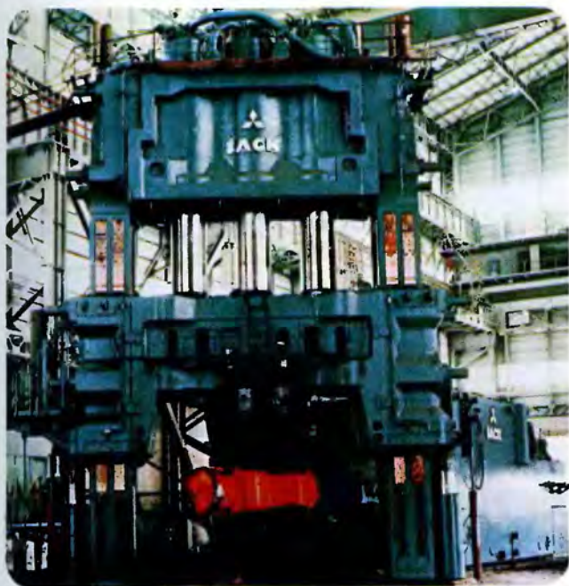
Кузнечные прессы с силой сжатия 120 мн (12 000 кгс) .
