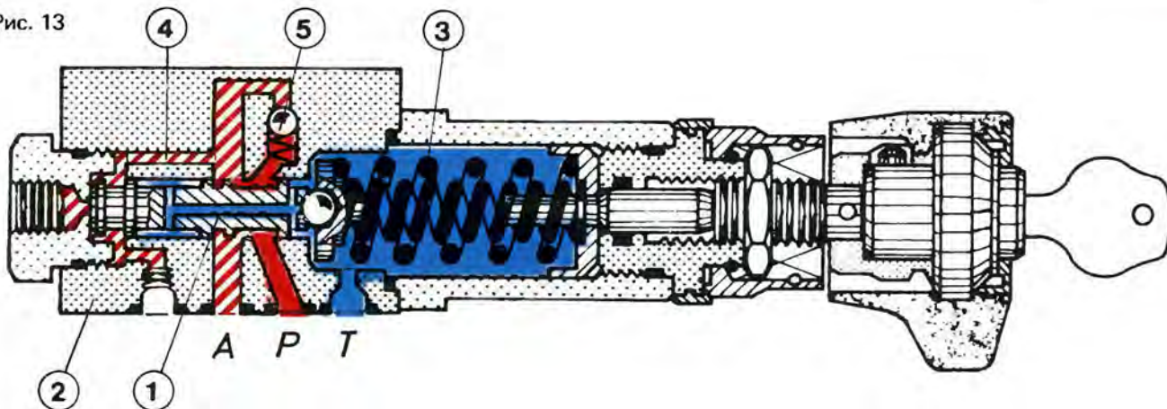
Редукционный клапан тип DR 6 D в разрезе
