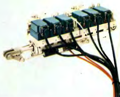
Сдвоенная-триплексная-мажоритарная система
