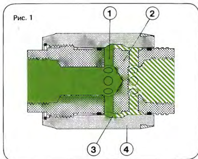
Простой дроссельный клапан, тип MG
