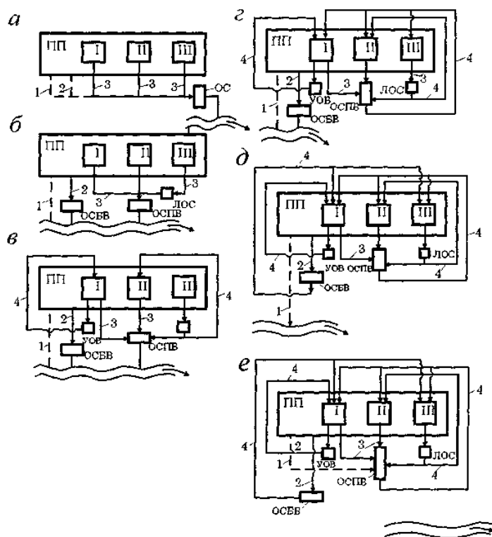
Рис.3.4. Системы водоотведения промышленных предприятий:
