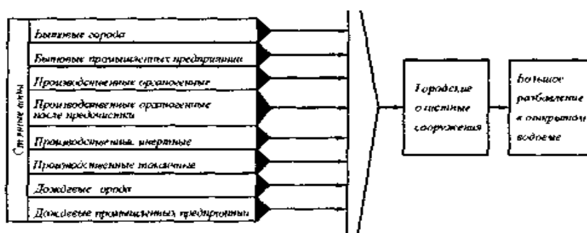
Рис.3.5. Граф возможных вариантов водоотведения для общесплавной системы
