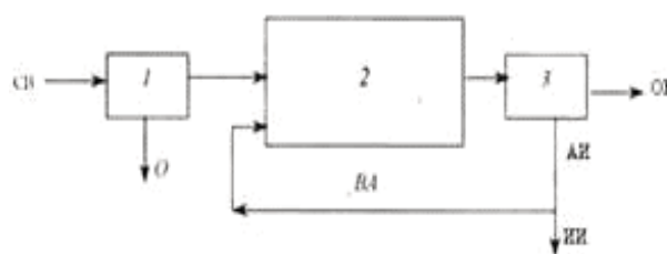
Рис. 7.4. Технологическая схема очистной станции с биологической очисткой сточных вод на аэротенках
