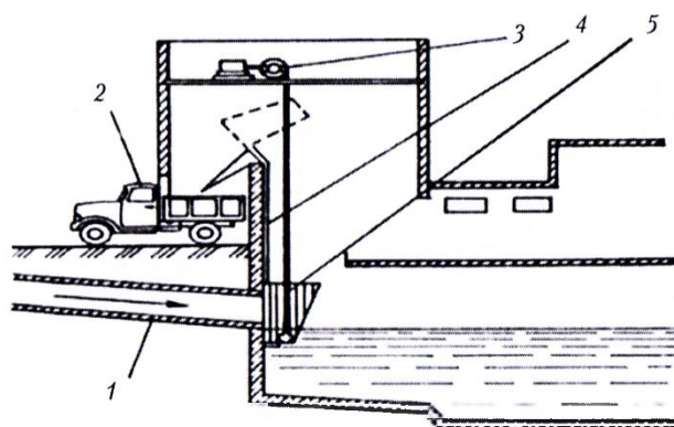
Рис. 7.24. Контейнерный способ отделения крупных включений из жидкого навоза: 1 – навозопровод; 2 – автосамосвал; 3 – лебедка; 4 – направляющие; 5 – решетчатый контейнер
