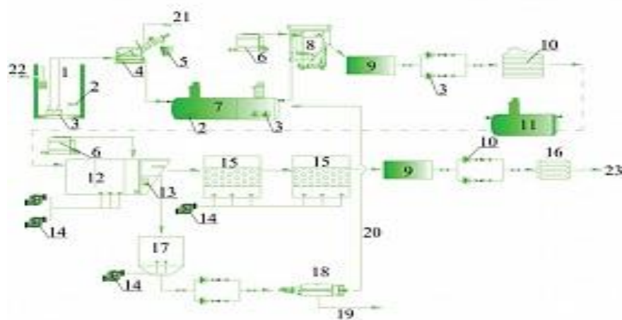
Рис. 7.25. Комплекс оборудования для очистки сточных вод
