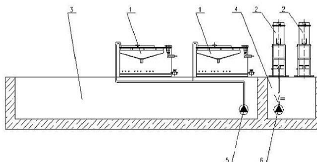
Рис. 7.10. Технологическая схема очистки ливневых стоков.
