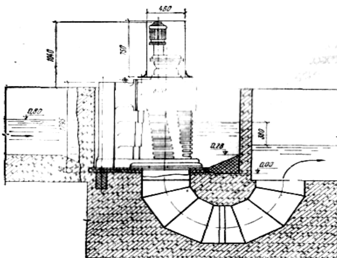
Рис. 7.15. Схема установки решетки-дробилки РД-600.
