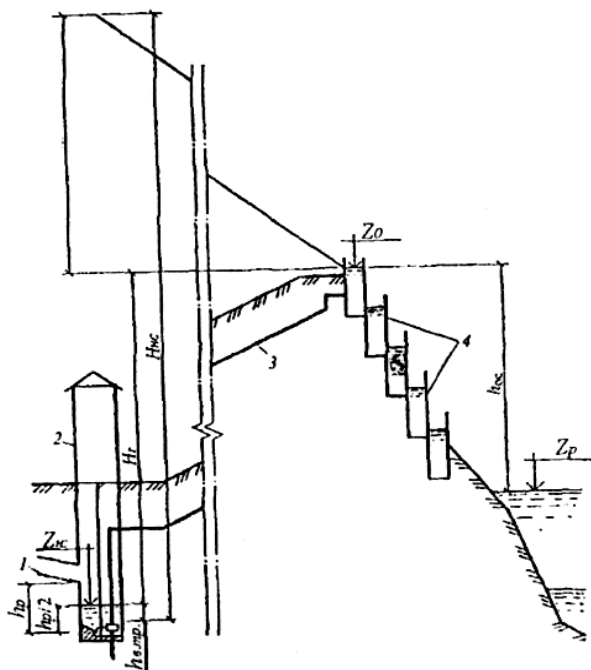
Рис.6.2. Высотная схема расположения насосной станции и напорного трубопровода: 1 – самотечный подводящий трубопровод; 2 – насосная станция; 3 – напорный трубопровод; 4 – очистные сооружения.
