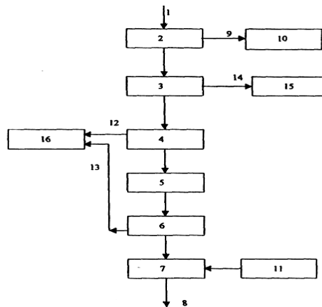
Рис. 7.3. Технологическая схема очистной станции с биологической очисткой сточных вод на биофильтрах:
