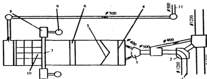
Рис. 5.3. Очистные сооружения камерного типа:
