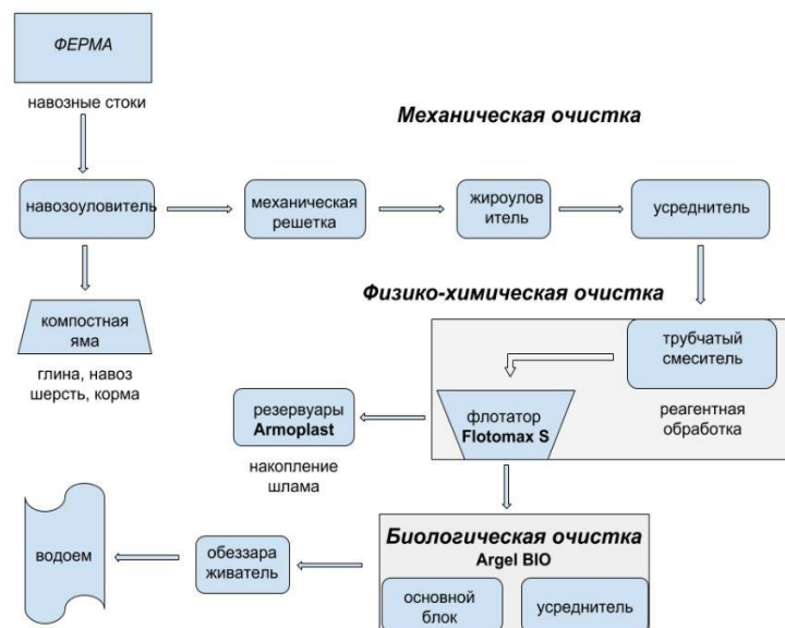
Рис. 7.13. Схема очистки сточных вод животноводческого комплекса
