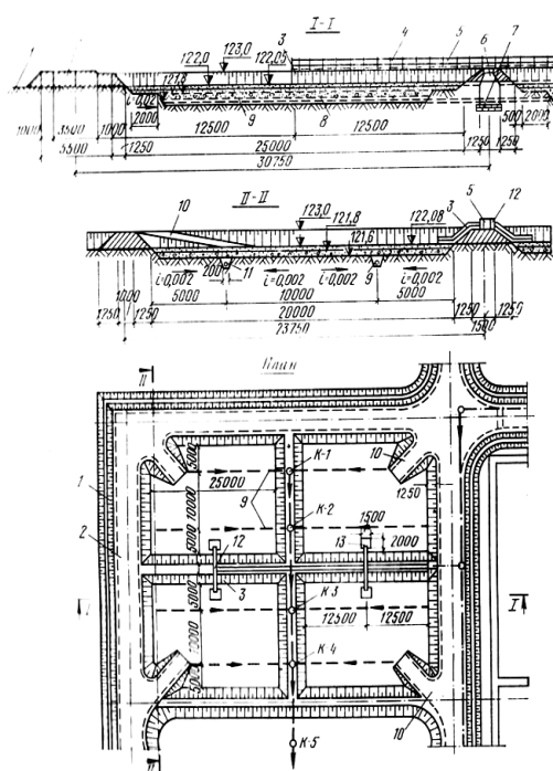
Рис.7.19. Иловые площадки:
