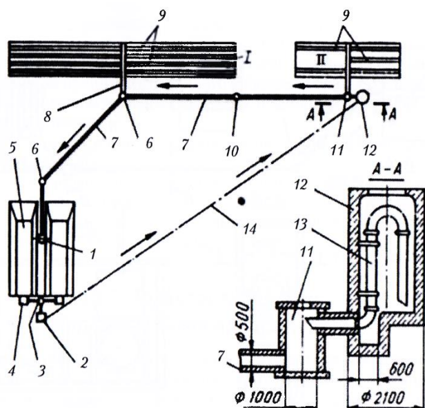
Рис. 7.23. Схема расположения безнапорного навозопровода на свиноводческой ферме на 1200 голов: I – откормочник; II – маточник; 1 – распределительная камера; 2 – насосная станция; 3 – жижеборник; 4 – камера фильтрации; 5 – навозохранилище; 6 – поворотный колодец; 7 – наружный навозопровод; 8 – поперечный канал; 9 – продольные каналы; 10 – линейный смотровой колодец; 11 – узловой колодец; 12 – промывочный колодец; 13 – сифонное устройство; 14 – напорный жижепровод
