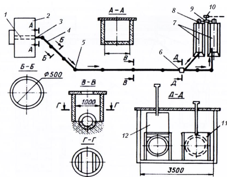
Рис. 7.22. Схема безнапорного навозопровода на ферме по откорму КРС на 1 тыс. голов: 1 – поперечный канал откормчика; 2 – здание; 3 – наружный канал; 4 – навозопровод; 5 – смотровые и поворотные колодцы; 6 – распределительная камера; 7 – навозохранилища; 8 – камера фильтрации; 9 – жижеборник; 10 – насосная станция; 11 и 12 – задвижки
