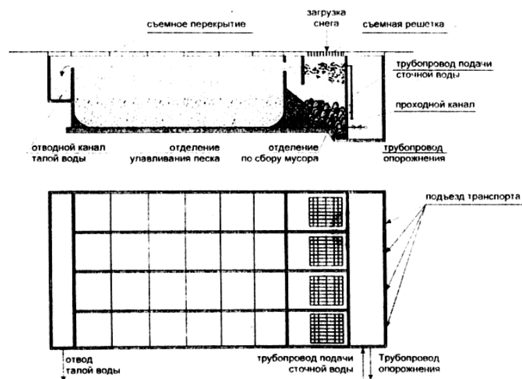
Рис. 4.6. Снегосплавная камера с улавливанием песка и крупных включений.
