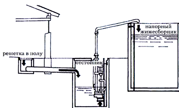
Рис. 7.20. Линия сбора сточных вод из помещения с животными
