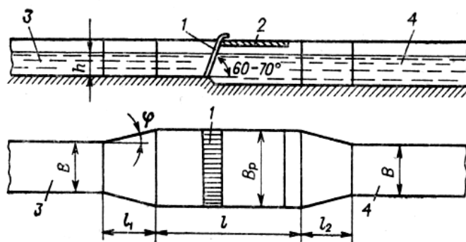
Рис. 7.14. Схема решетки простейшего типа:
