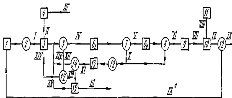
Рис. 7.26. Схема биологической очистки навозных сточных вод на свиноводческих комплексах:
