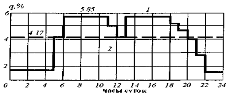
Рис. 4.1. Ступенчатый график притока сточных вод.
