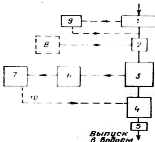
Рис.7.1. Схема станции с механической очисткой сточных вод 1 – решетка; 2 – песколовка; 3 – отстойники; 4 – хлораторная; 5 – контактный резервуар; 6 – метантенк; 7 – иловые площадки; 8 – песковые площадки; 9 – дробилки; 10 – трубопровод дренажной воды
