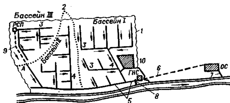
Рис. 3.1. Общая схема водоотведения населенного пункта.
