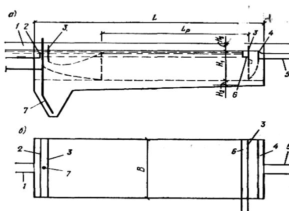
Рис. 7.18. Горизонтальный отстойник
