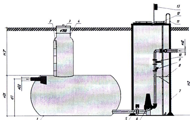
Рис. 7.21 КНС с аккумулярующим резервуаром и сухой приемной камерой: 1 – корпус приемного резервуара; 2 – лестница; 3 – крышка с воздухоотводом; 4 – технологический лаз; 5 – затвор; 6 – насос; 7 – корпус КНС; 8 – площадка обслуживания; 9 – обратный клапан; 10 – задвижка; 11 – поручень; 12 – крышка с технологическими лазами; 13 – щит управления
