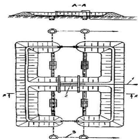
Рис. 7.17. Песковая площадка: 1 – пескопровод; 2 – разводящий лоток; 3 – трубопровод для отвода дренажной воды.
