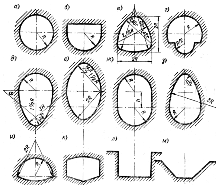
Рис. 4.3. Формы поперечного сечения водоотводящих труб, коллекторов и каналов: а – круглое; б – полукруглое; в – шатровое; г – банкетное; д – яйцевидное (овоидальное); е – эллиптическое; ж – полукруглое с прямыми вставками; з – яйцевидное перевернутое; и – лотковое; к – пятиугольное; л – прямоугольное; м – трапецидальное.
