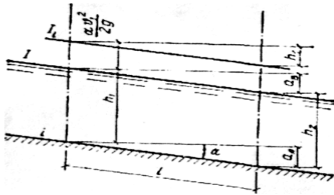
Рис.4.2. Схема безнапорного режима движения потока.
