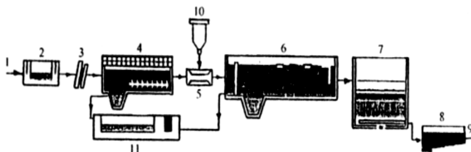
Рис. 5.4. Принципиальная схема очистки промышленного ливневого стока на МГУП «Промотходы»: 1 – поступающий на очистку сток; 2 – приемная камера; 3 – механизированные решетки; 4 – песколовки; 5 – смеситель; 6 – горизонтальные отстойники; 7 – мелкозернистые фильтры; 8 – резервуар чистой воды; 9 – сброс очищенного стока в водоприемник; 10 – реагентное хозяйство; 11 – бетонированные площадки для переработки нефтесодержащих осадков.
