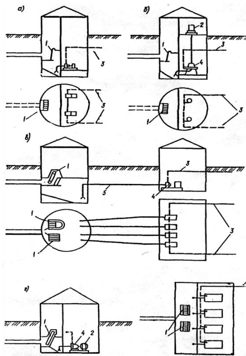
Рис.6.1. Схемы насосных станций:
