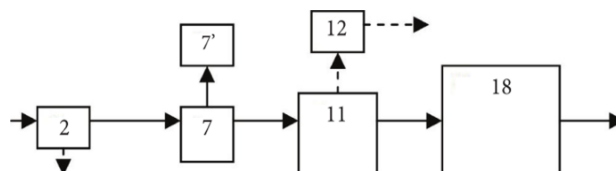
Рис. 7.2. Схема станции с биологической очисткой сточных вод в естественных условиях 1 - сточные воды; 1' - очищенные сточные воды; 2 - решетки; 3'- отбросы с решеток на почвенное обезвреживание; 7 - песколовки; 7' - песковые площадки; 11 - первичные отстойники; 12 - сооружения для переработки и обезвреживания осадков; 12' - на утилизацию в качестве удобрения; 18 - поля орошения или поля фильтрации
