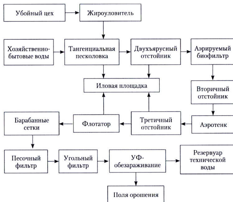
Рис. 7.8. Принципиальная схема очистки сточных вод птицефабрики с полной биологической очисткой
