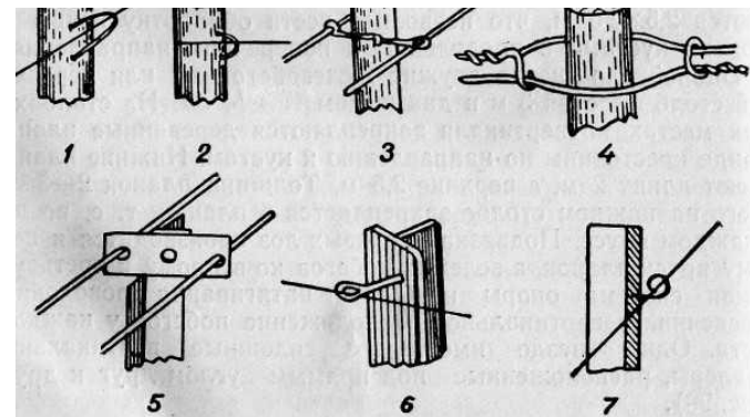
Рис. 101. Способы укрепления проволоки.
