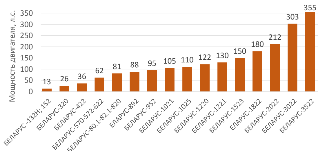
Рис. 1.1. Мощность двигателей тракторов «Беларус»
