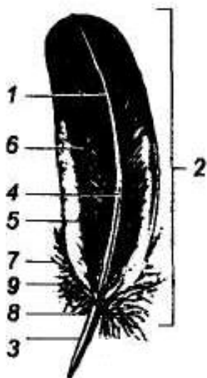
Рис. 10. Строение перьев:
