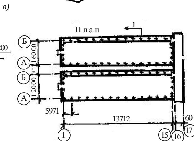
Рисунок 7.8 – Теплицы зимние ангарного типа: а – общий вид; б – разрез; в – план
