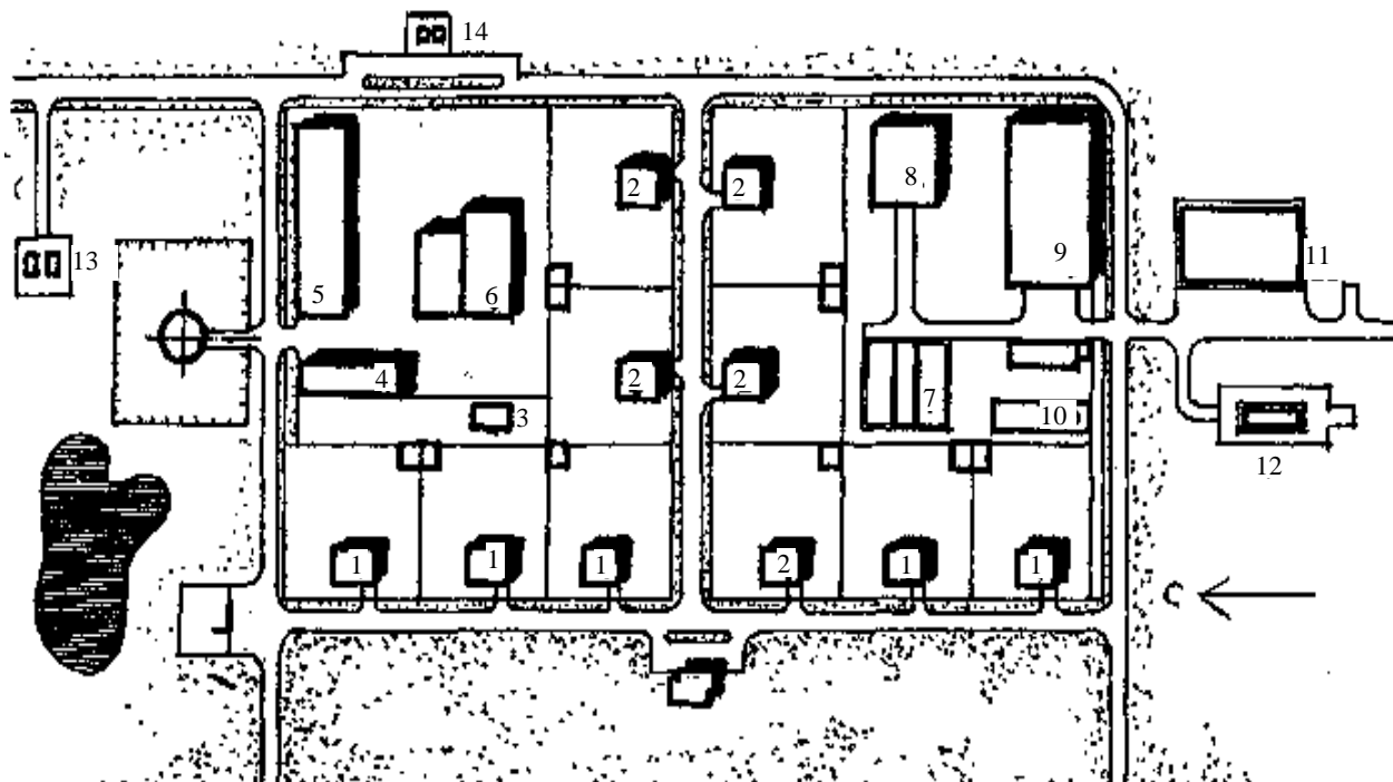
Рисунок 7.13 – Генплан фермерского хозяйства «Нива» Шкловского района:
